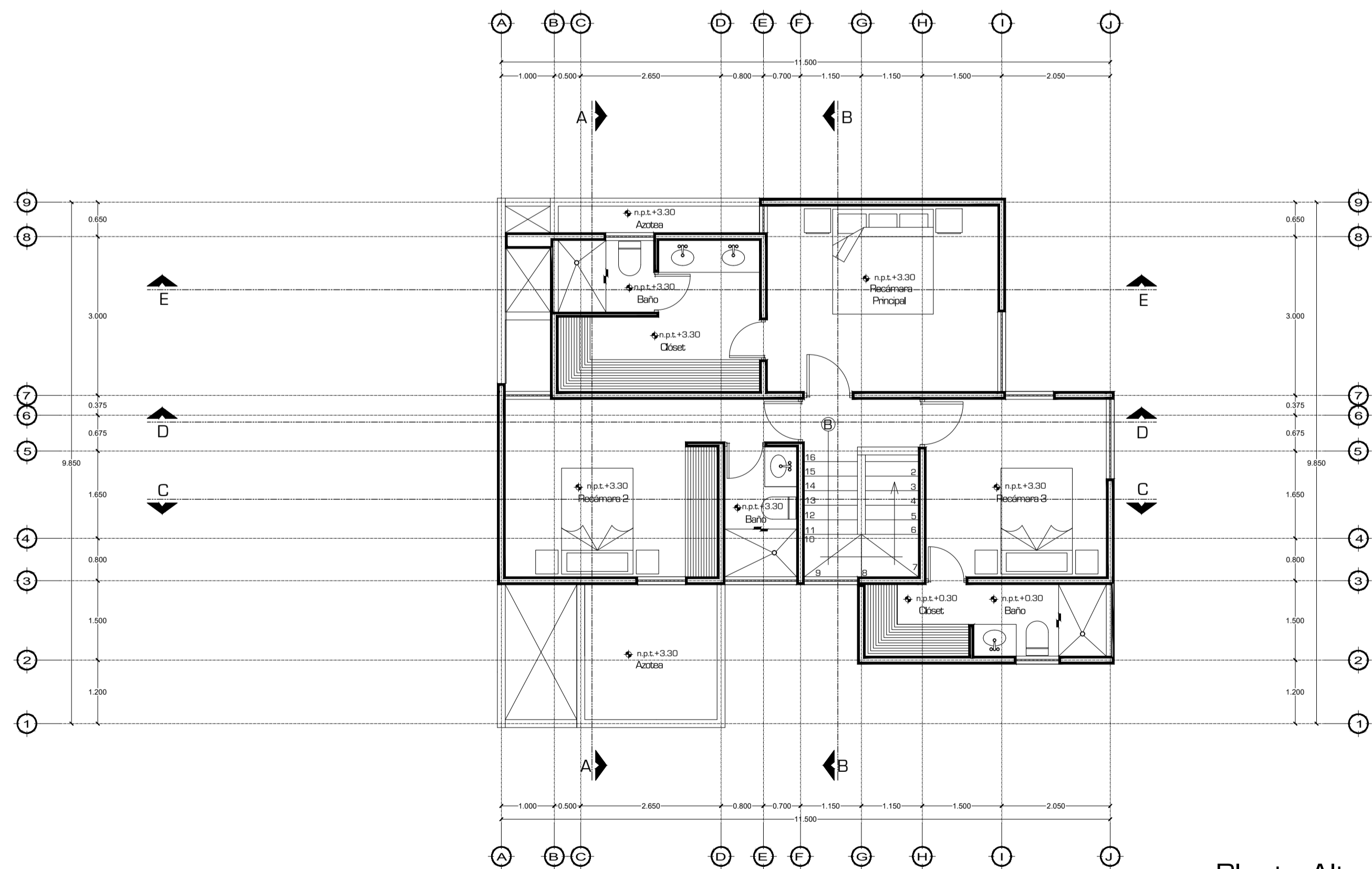
Planta Alta 81.19 m 2
