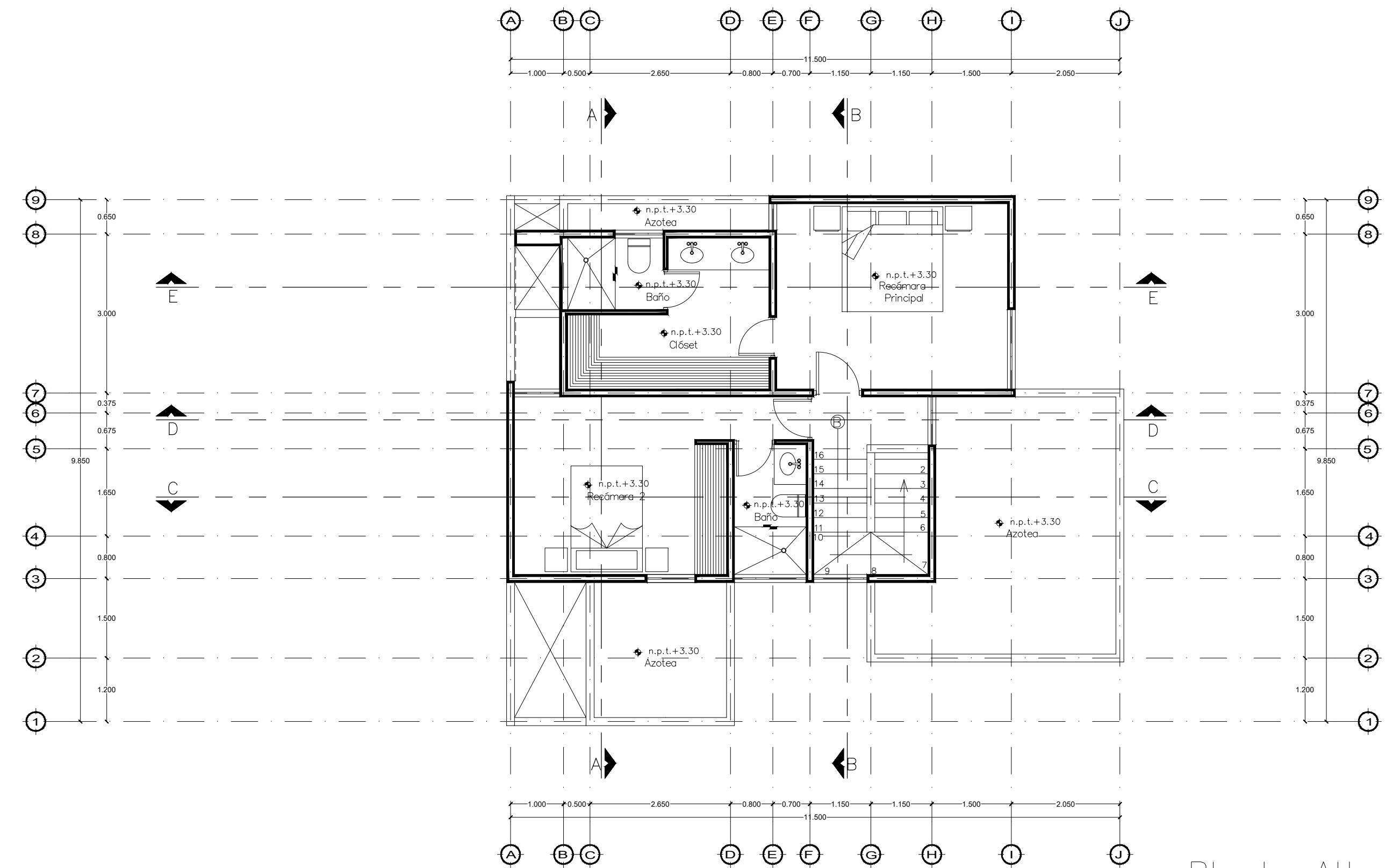
Planta Alta 61.18 m 2
