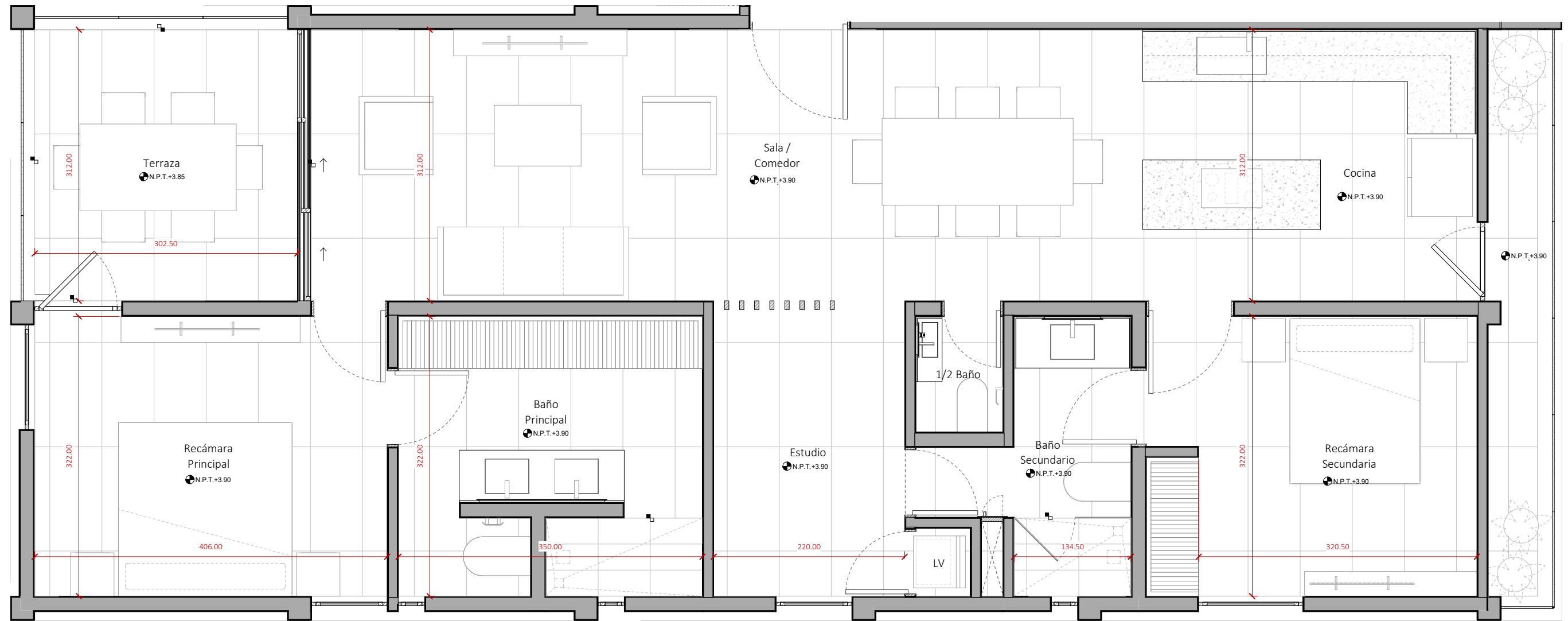
1 Nivel 01 - CHE DPTO A ESCALA 1 : 50
