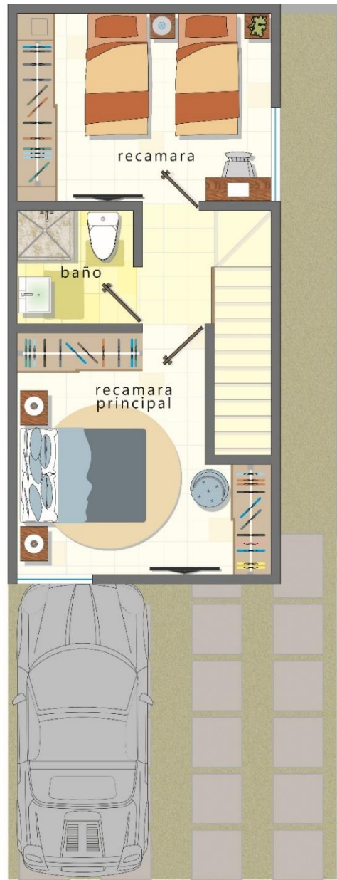
PLANTA ALTA
