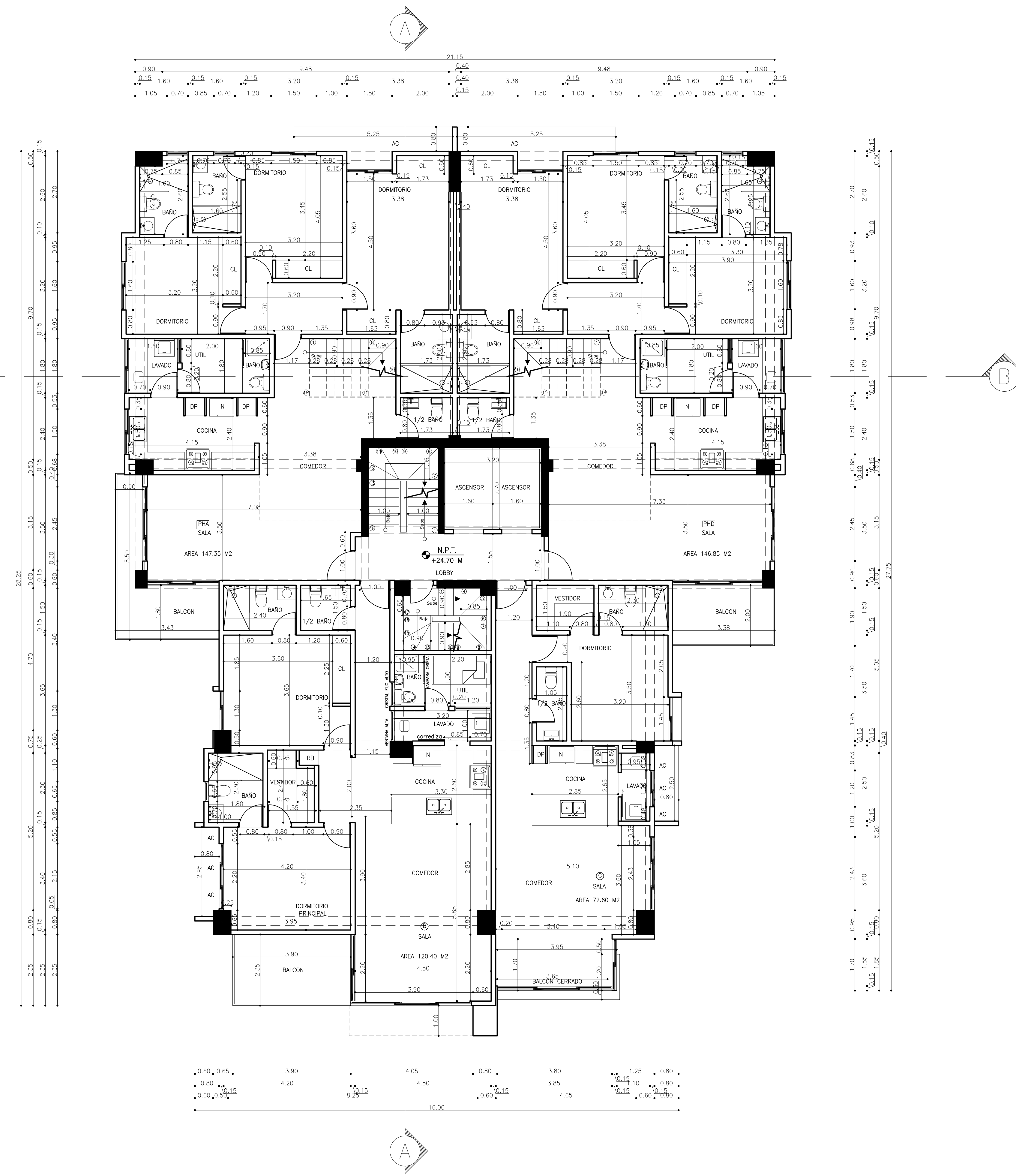
Planta Dimensionada 8vo
