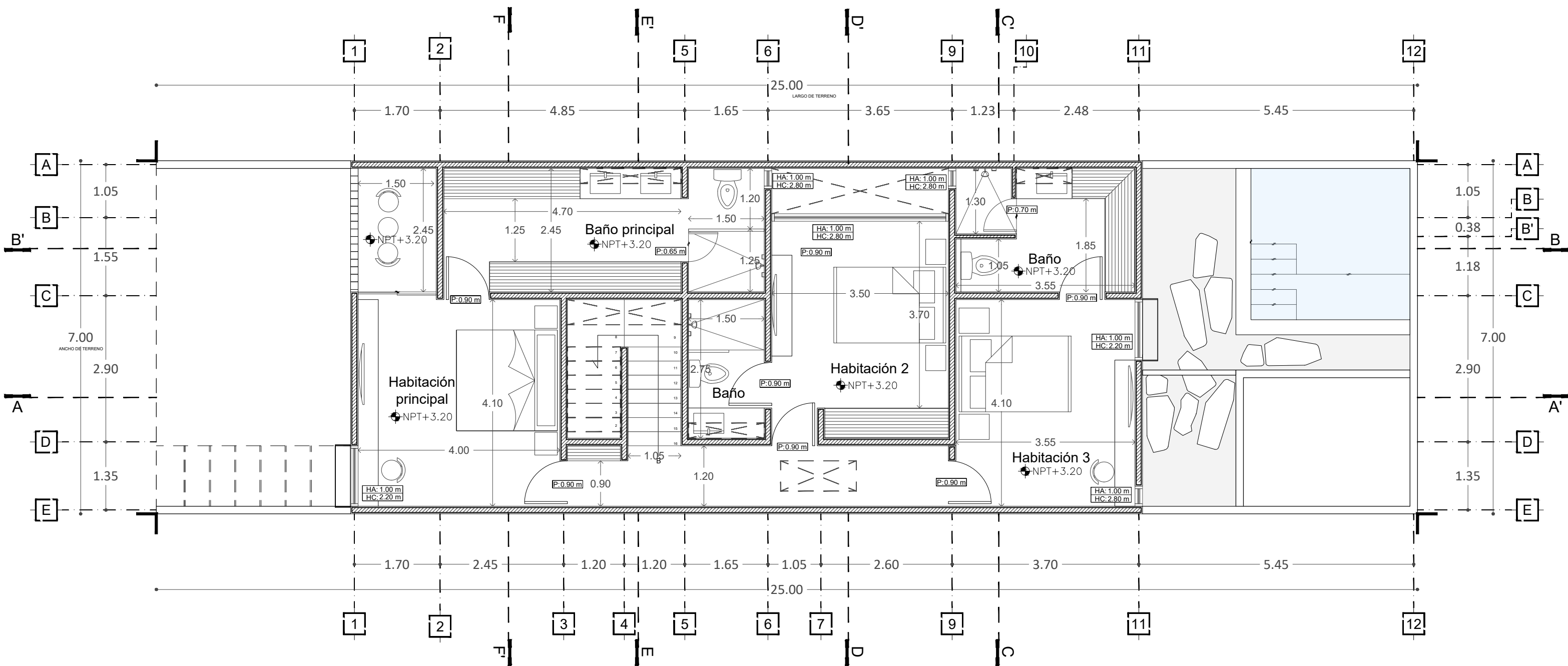
PLANTA ALTA
