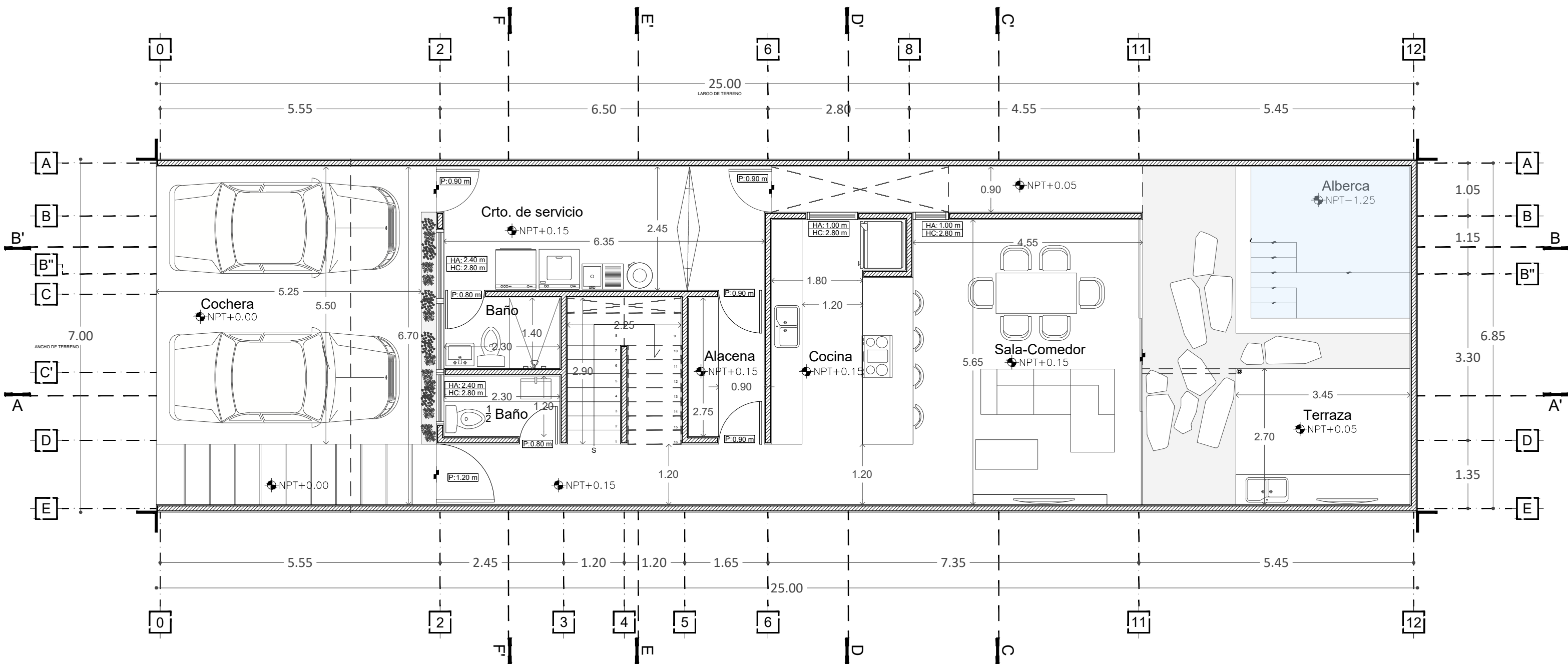
PLANTA BAJA
