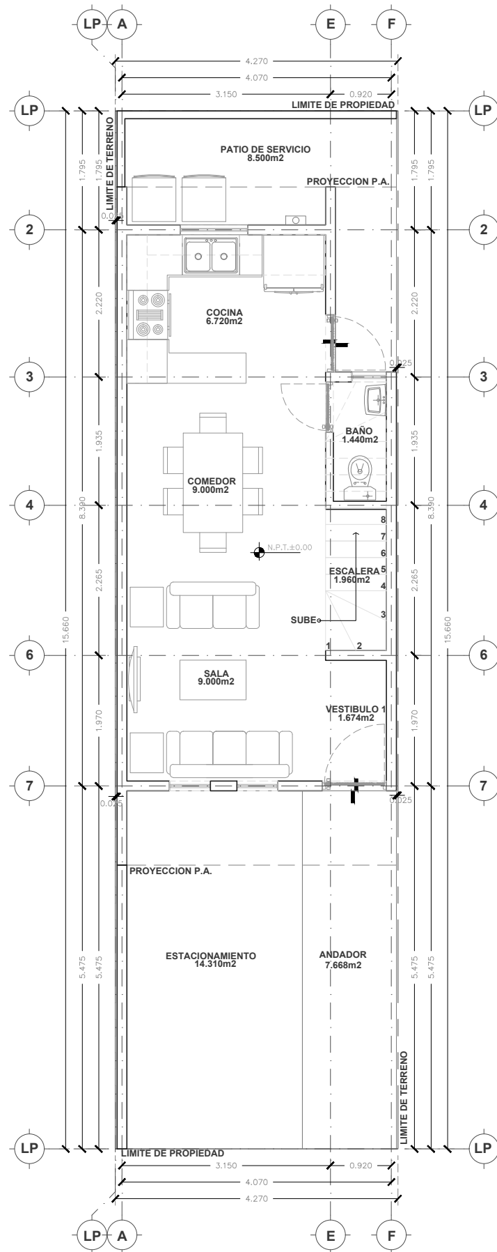
PLANTA BAJA
