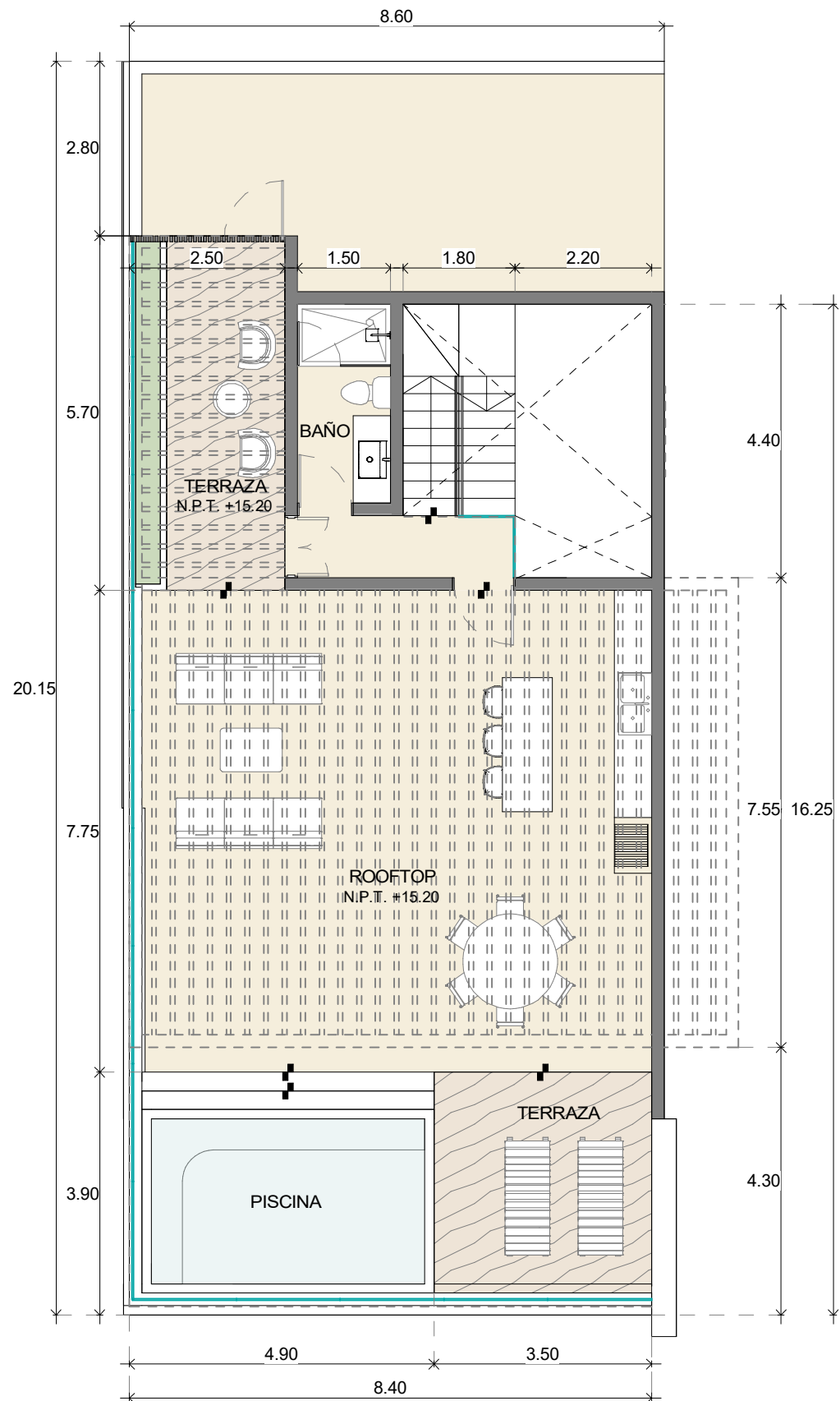
PLANTA ARQUITECTÓNICA ROOF TOP VILLA 1RT ESC- 1 : 100
