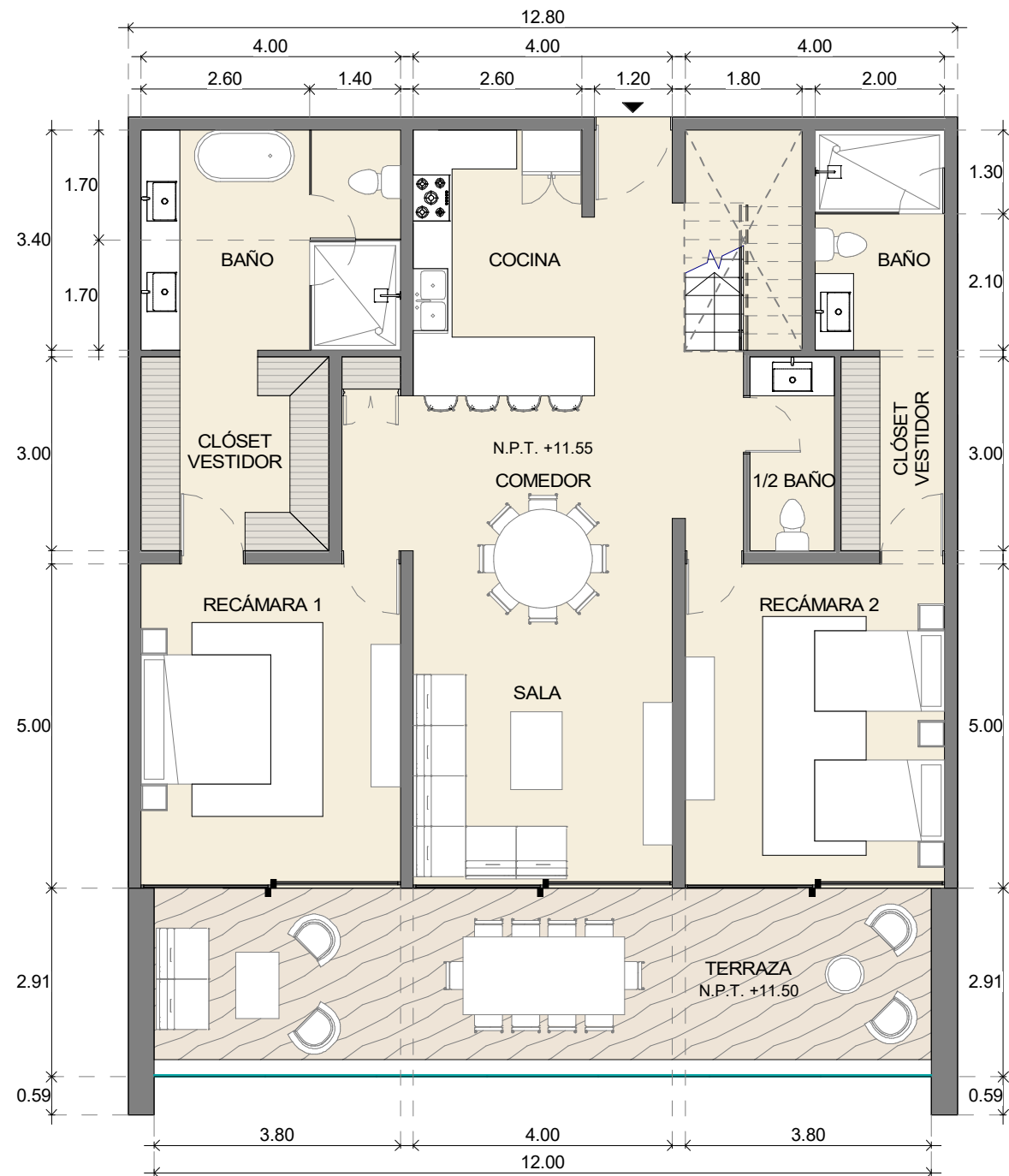
PLANTA ARQUITECTÓNICA BAJA VILLA 3RT
