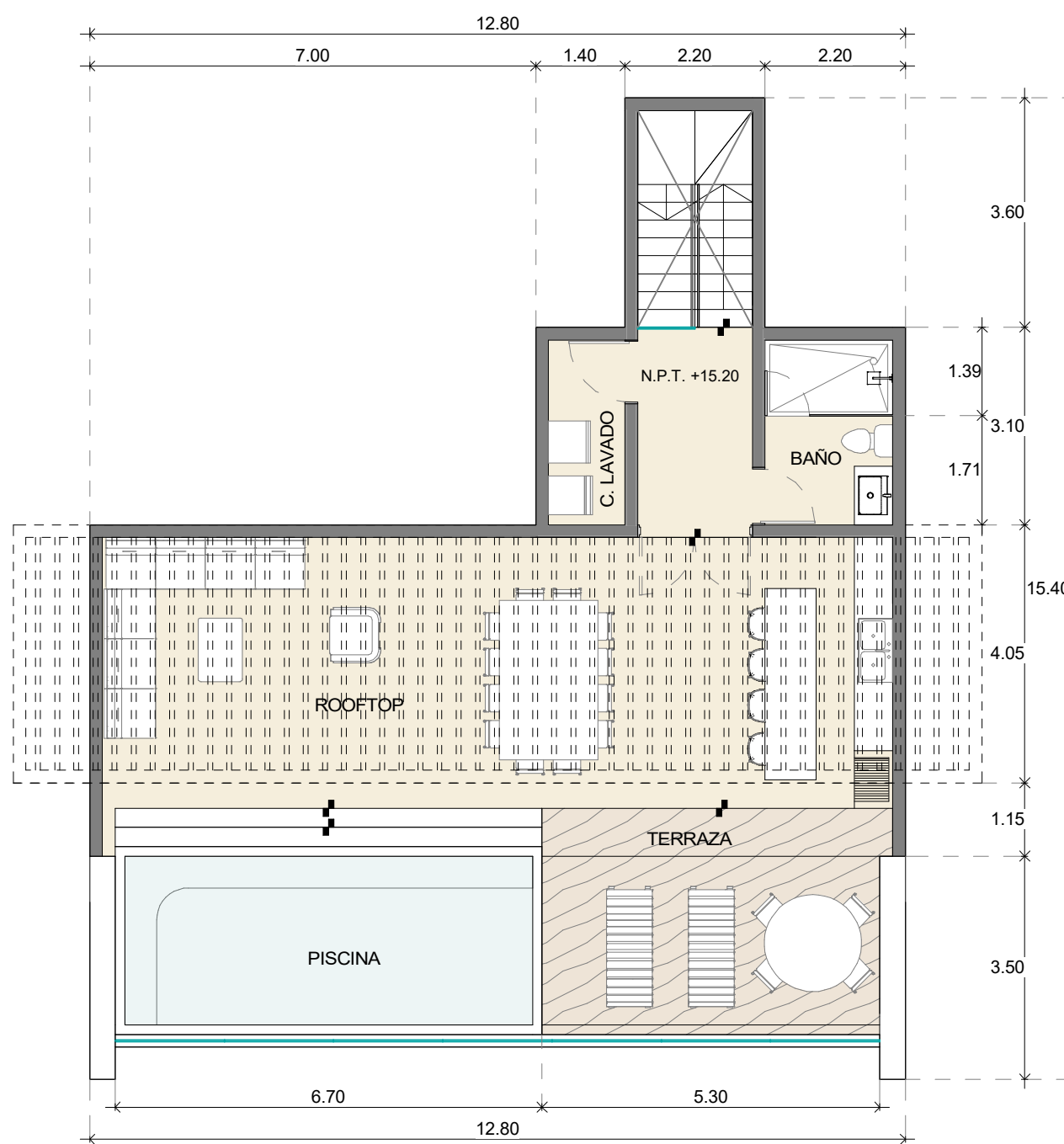
PLANTA ARQUITECTÓNICA ROOFTOP VILLA 3RT
