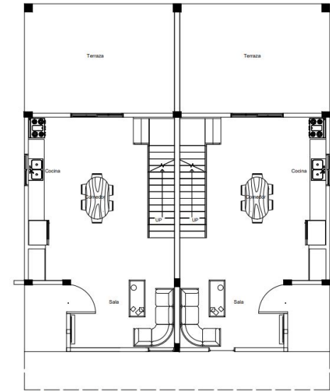
PLANTA ARQUITECTÓNICA AMUEBLADA PRIMER NIVEL
