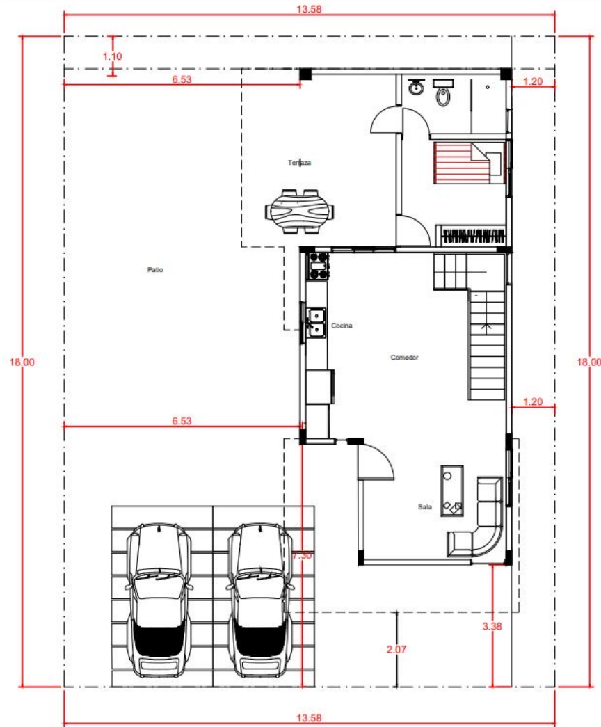
Planta Arquitectonica de Conjunto Victoria Plus 5ta etapa CV
