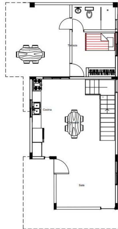
Planta Arquitectonica Amueblada Victoria Plus 5ta etapa CV
