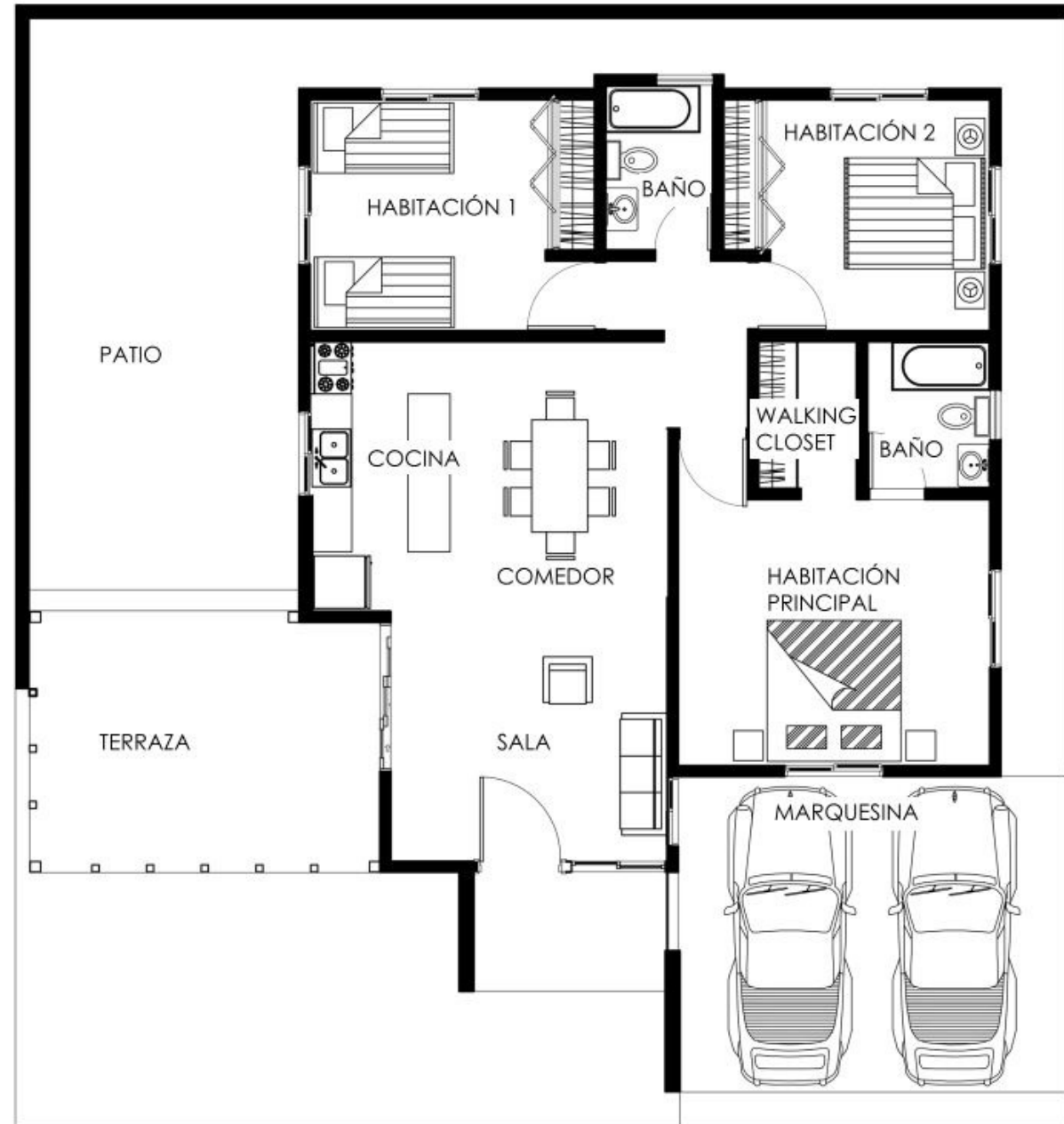
VILLA SARAI PLANTA ARQUITECTÓNICA AMUEBLADA
