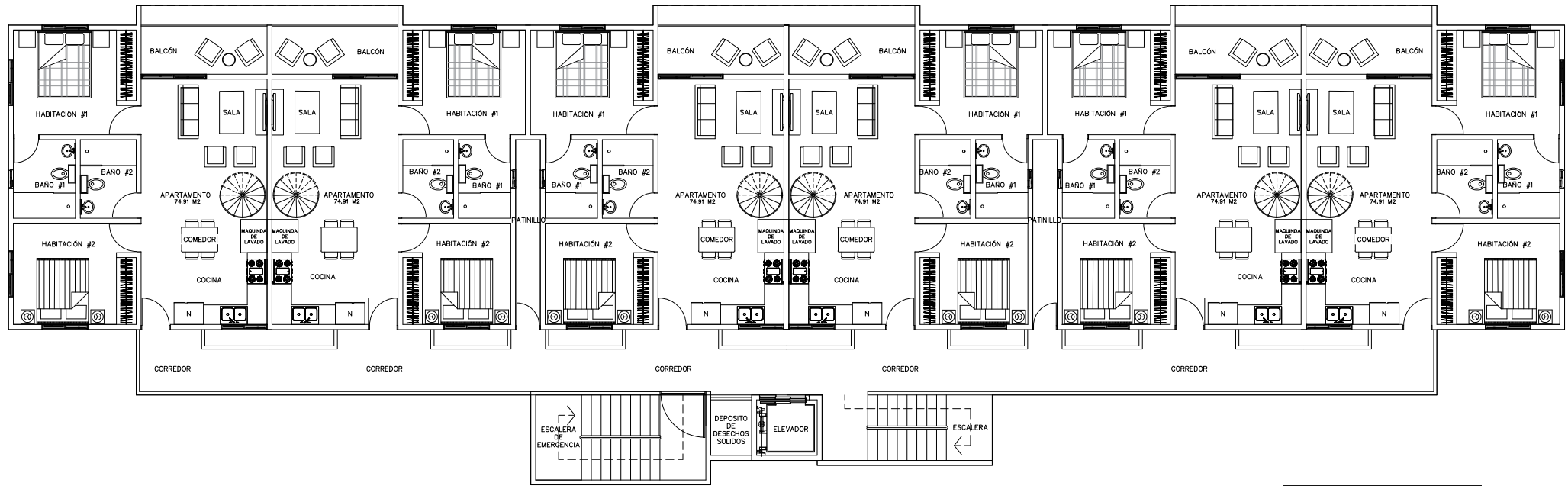
PLANTA ARQUITECTONICA AMUEBLADA CUARTO NIVEL TIPO A / 4 NIVELES
