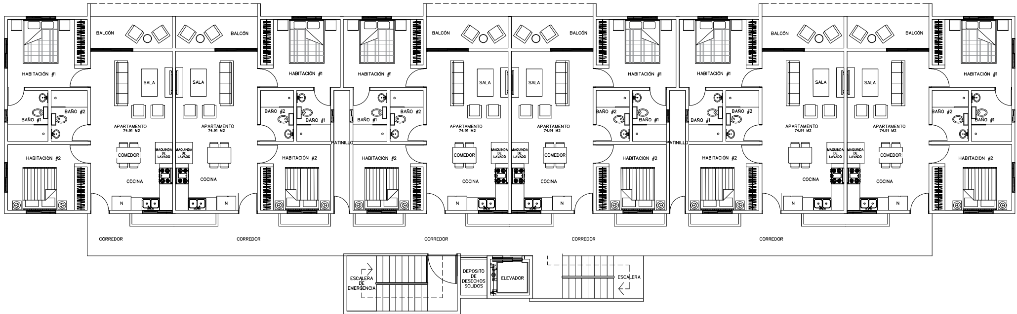
PLANTA ARQUITECTONICA AMUEBLADA PRIMER NIVEL TIPO A / 3 NIVELES
