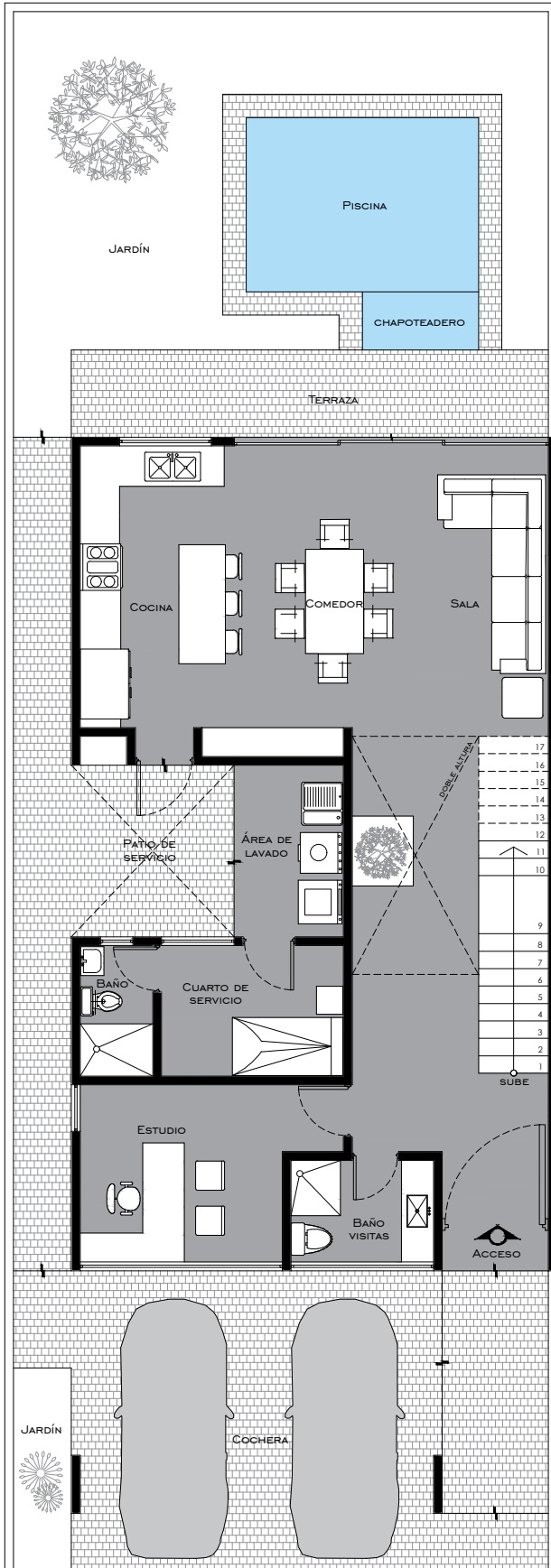
PLANTA BAJA
