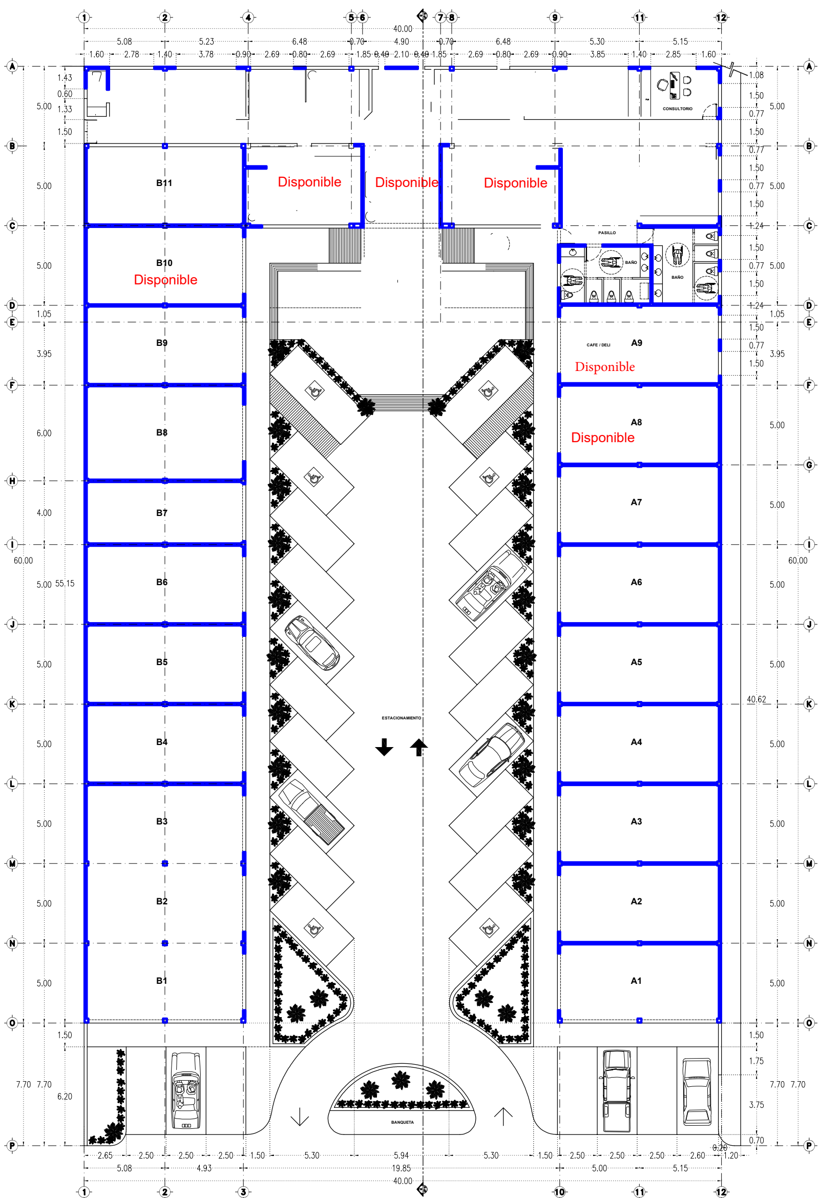
PLANTA ARQUITECTONICA BAJA 1:200
