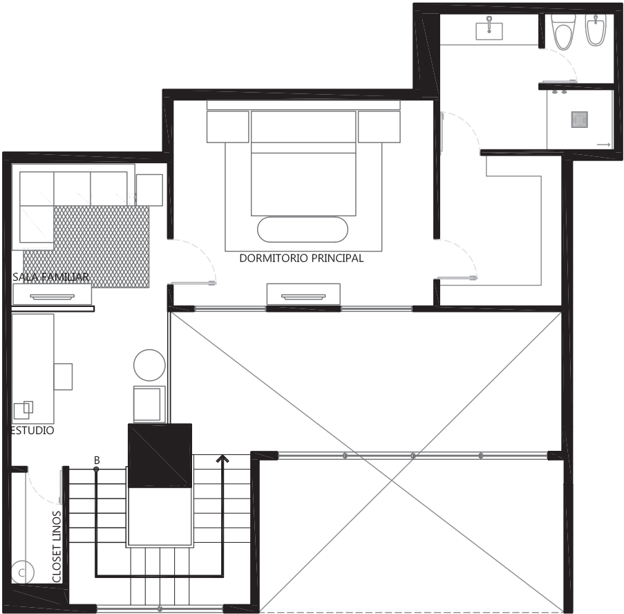
planta alta
