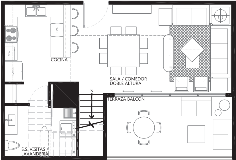
planta baja
