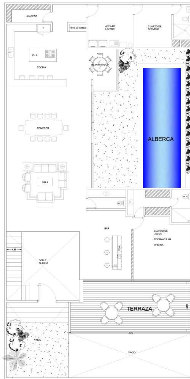
02 PLANTA ALTA PLANTA ARQUITECTONICA
