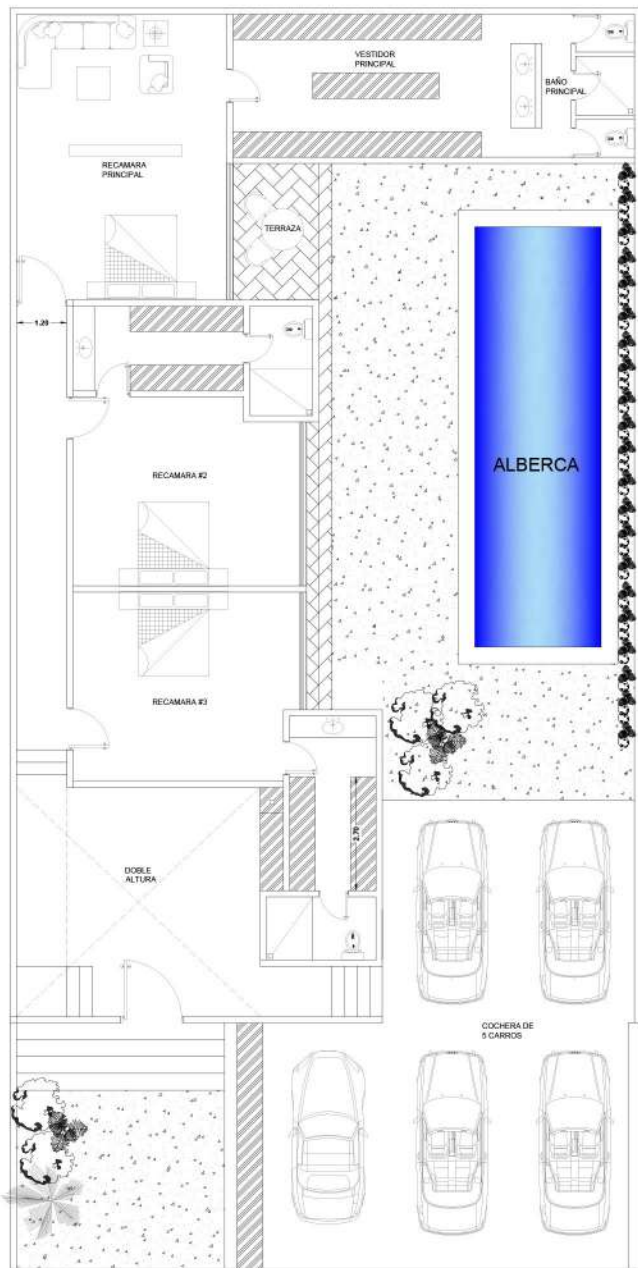
01 PLANTA BAJA PLANTA ARQUITECTONICA
