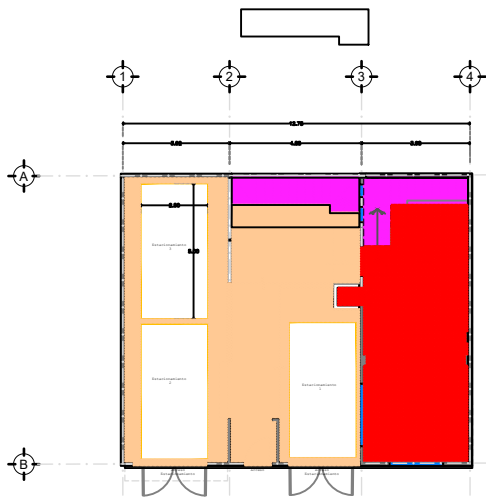
PLANTA ARQUITECTONICA PLANTA BAJA
