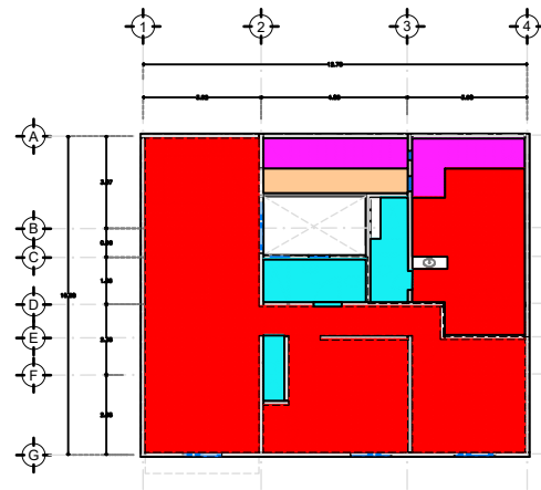
PLANTA ARQUITECTONICA 1N
