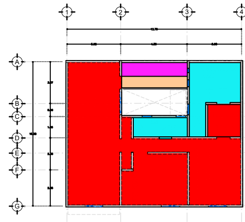
PLANTA ARQUITECTONICA 2N
