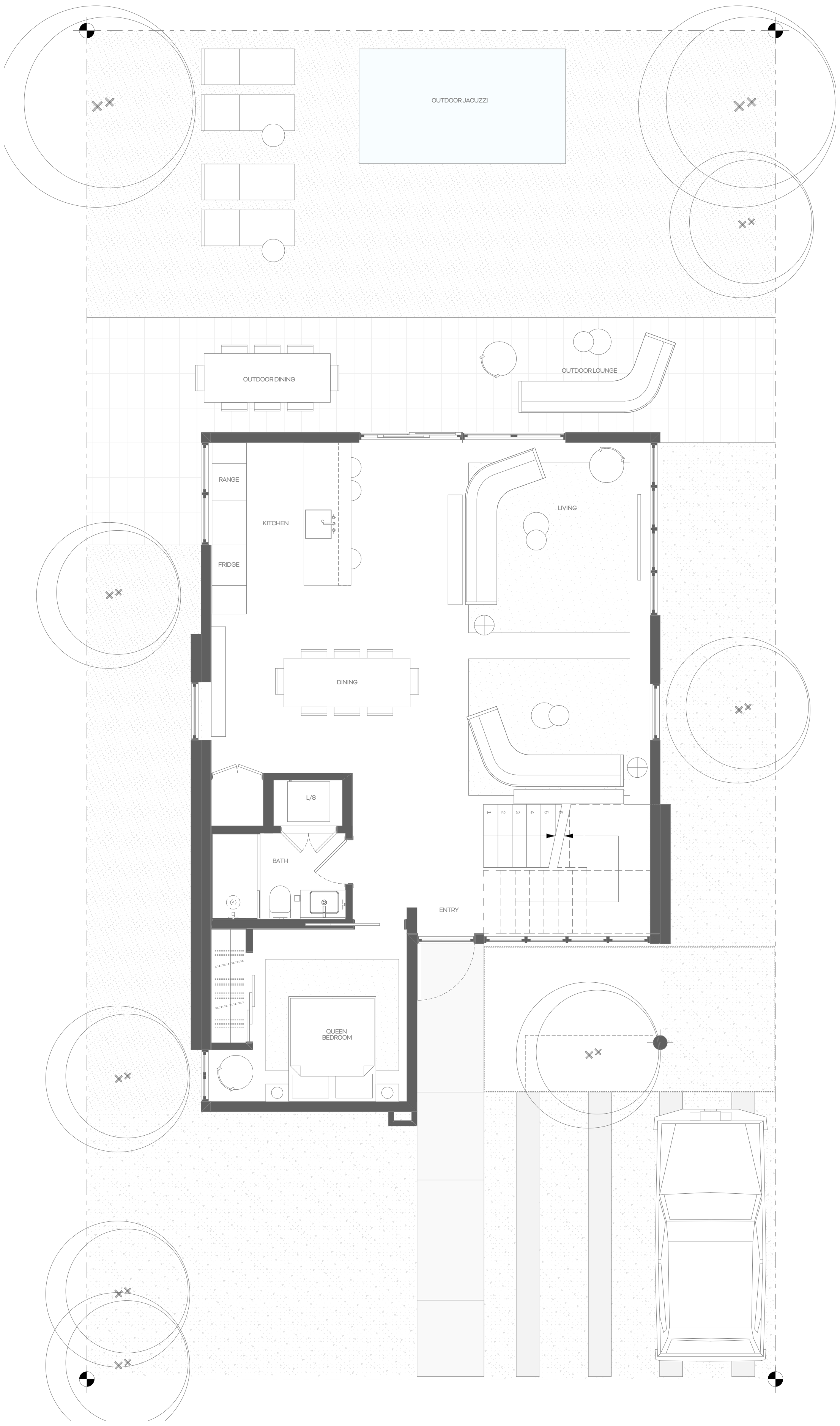
1. NIVEL 01 SCALE: 1:50
