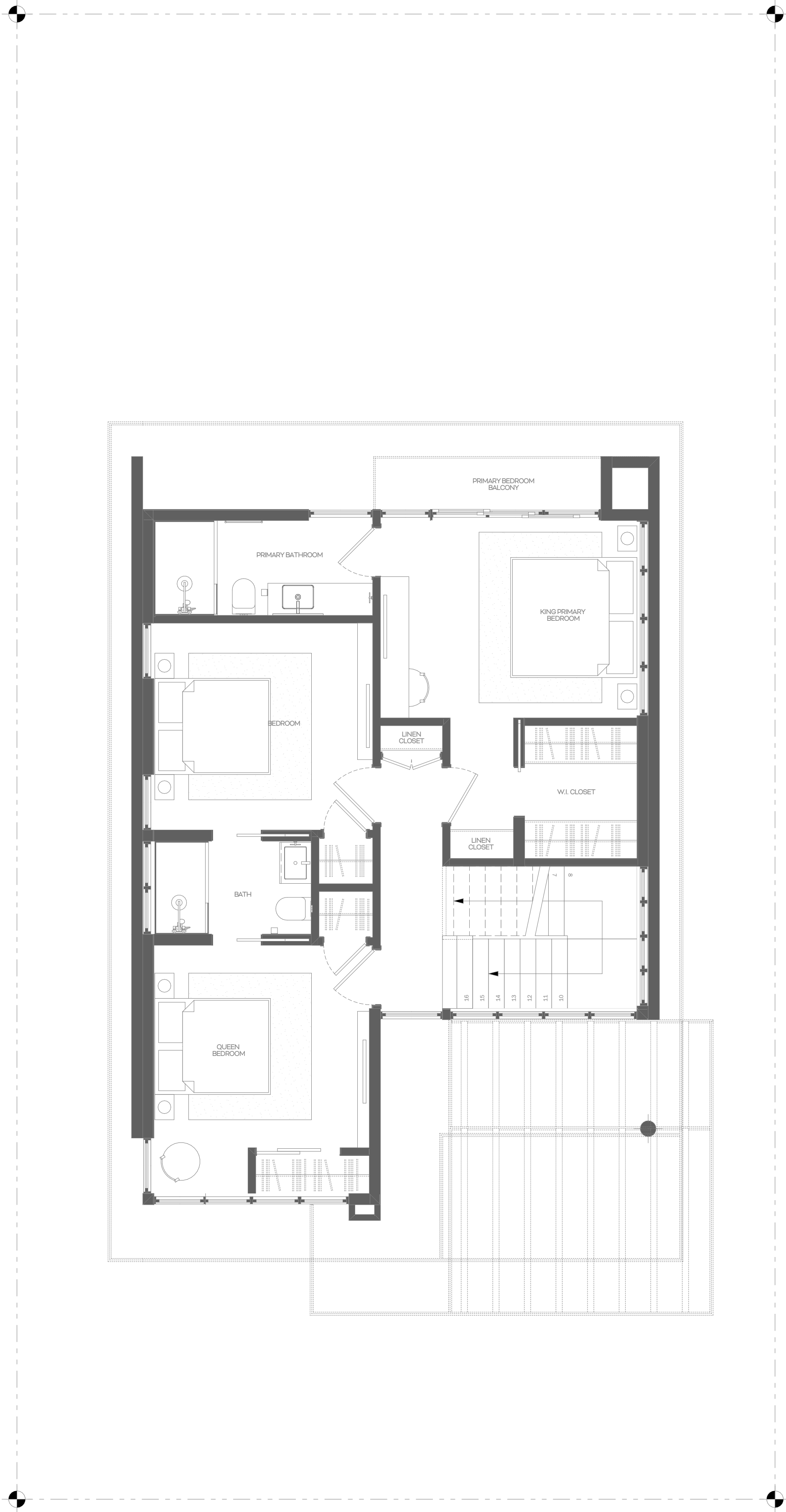
2. NIVEL 02 SCALE: 1:50
