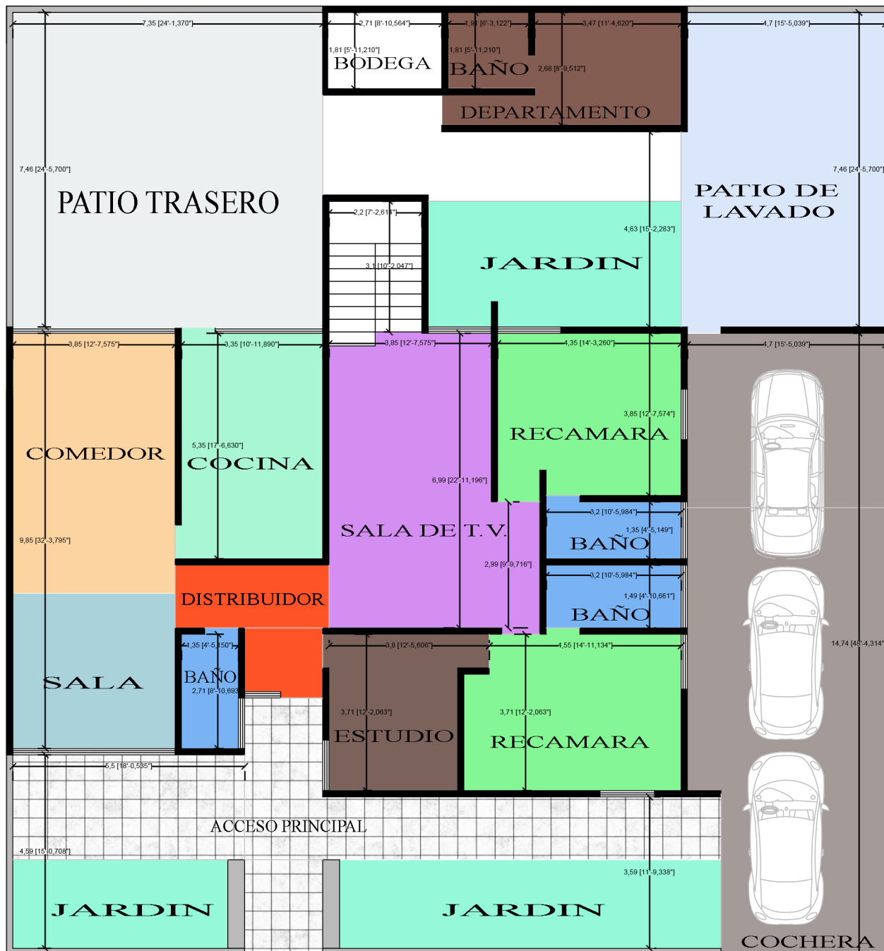
PLANTA ARQUITECTONICA BAJA.
