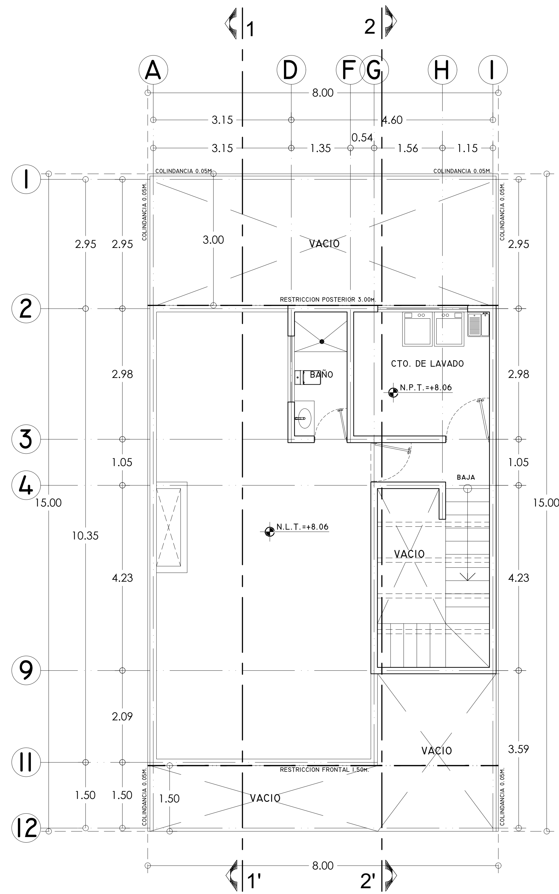
Planta 2do. Nivel.
