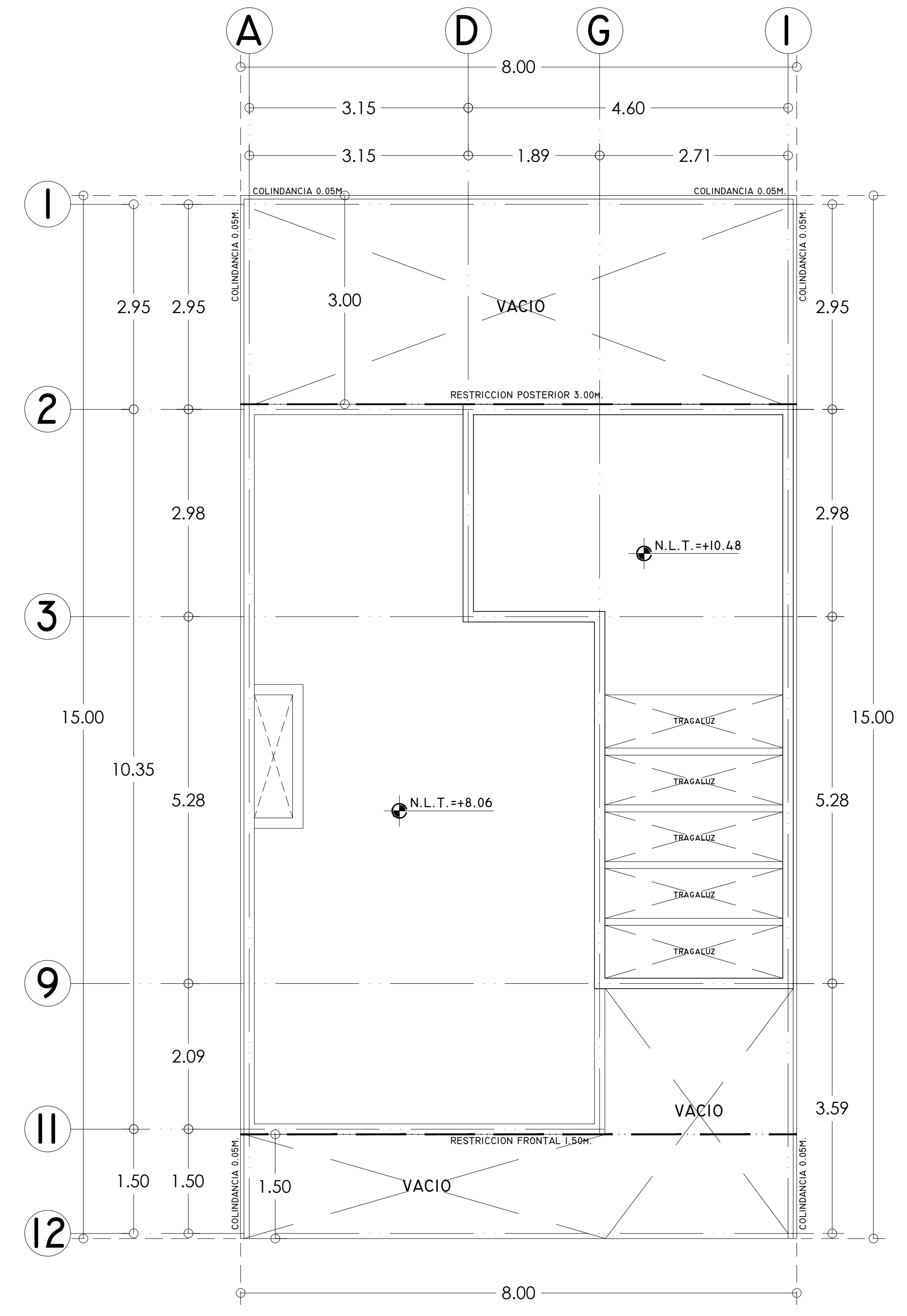
Planta Azotea.
