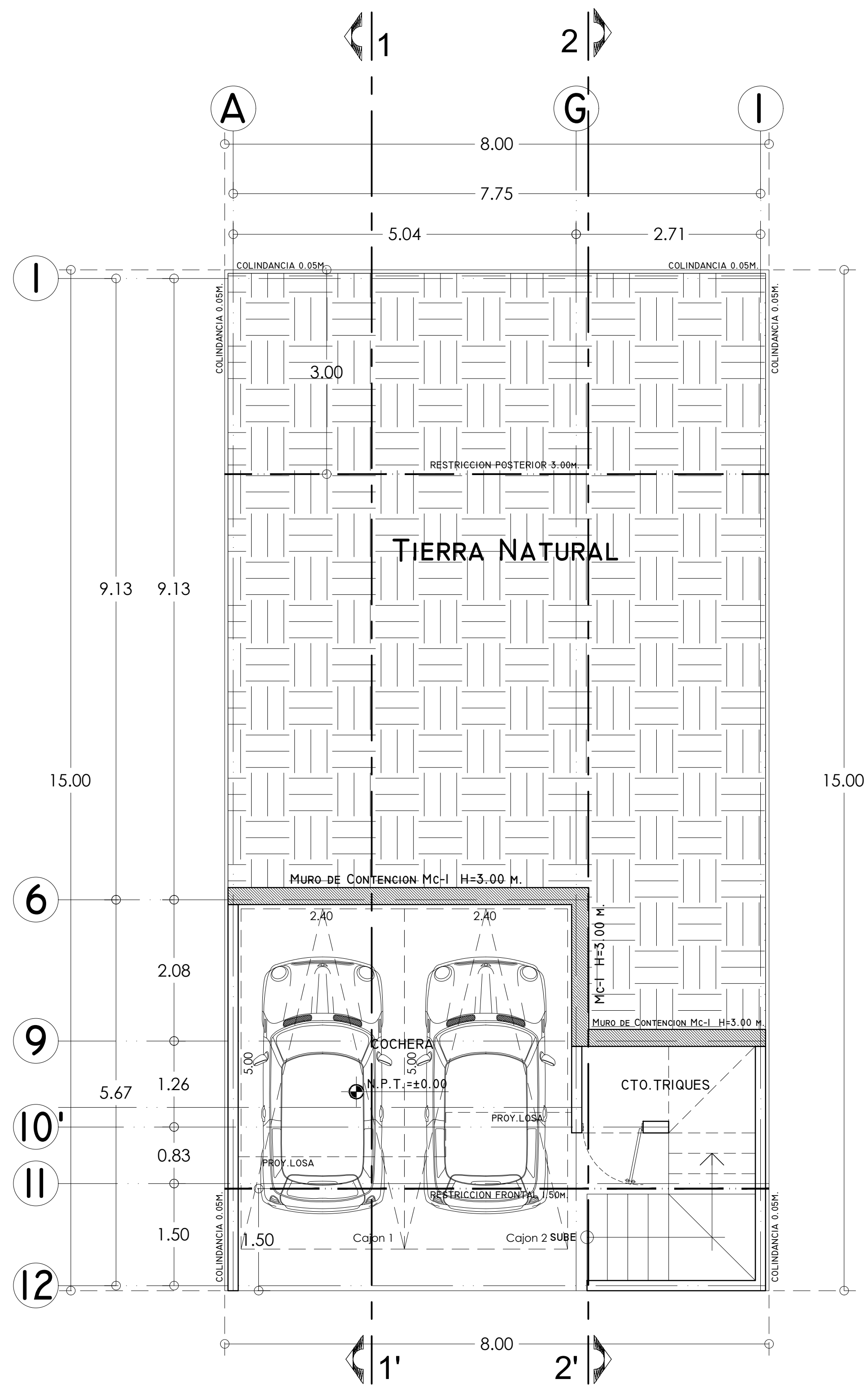
Planta Acceso.
