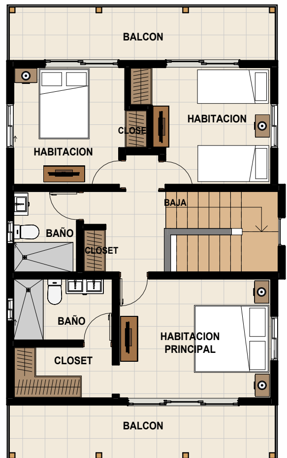
2 PLANO ARQUITECTONICO 2DO NIVEL 1 : 100
