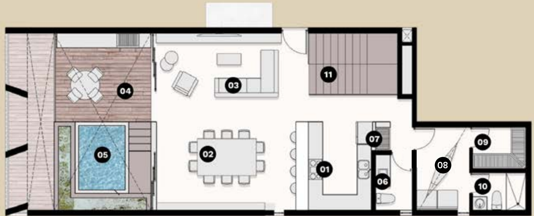
Planta Alta
