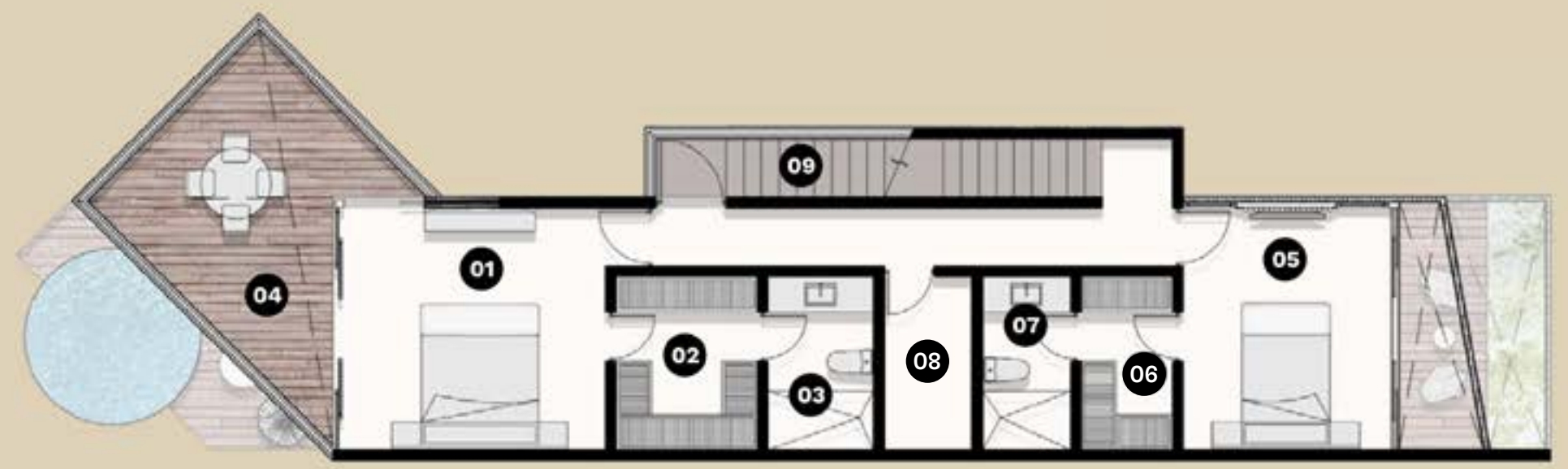
Planta alta
