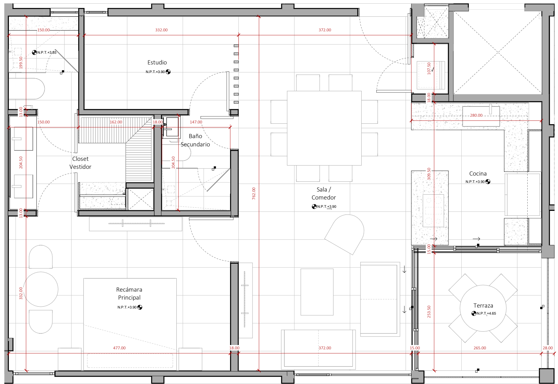
2 Nivel 01 - CHE DPTO B ESCALA 1 : 50
