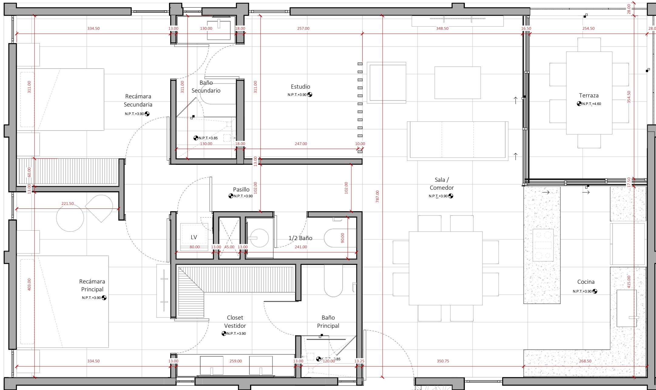
2 Nivel 01 - CHE DPTO D ESCALA 1 : 50
