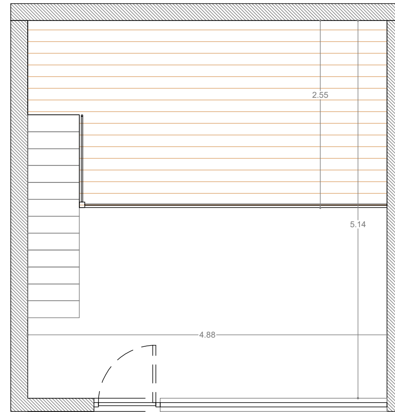
PLANTA ALTA 11.52 m 2
