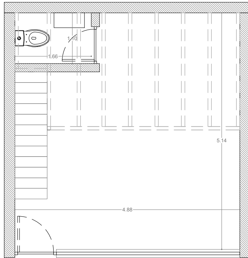
PLANTA BAJA 25.06 m 2
