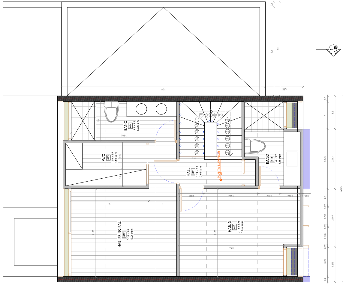
A1 Planta Dimensionada Casa Tipo B (Planta Alta) Scale: 1/25
