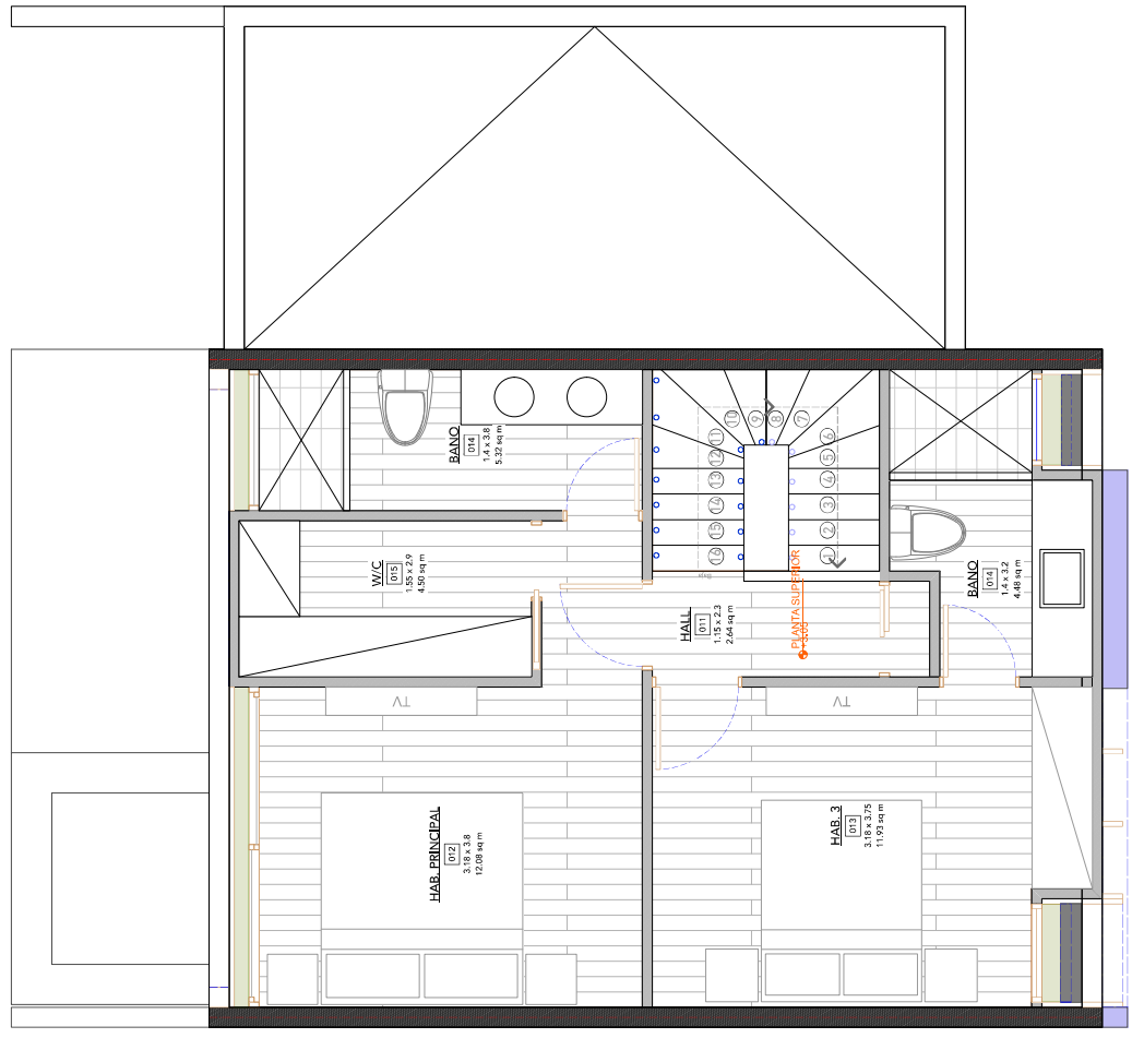
A1 | Planta Arquitectónica Casa Tipo B (Planta Alti)| Scale: 1/25
