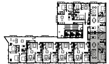
Planta Conjunto
