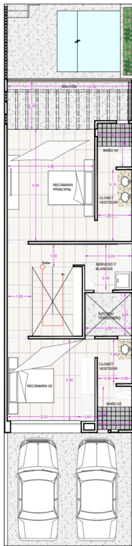
SEGUNDO NIVEL
