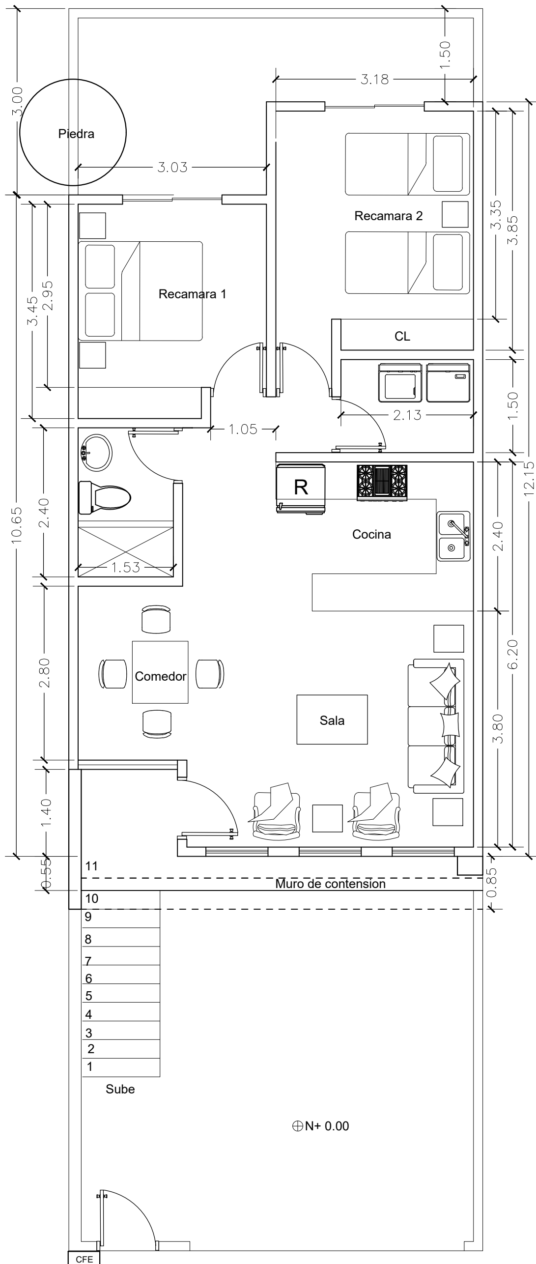
Planta Arquitectónica Escala 1:75
