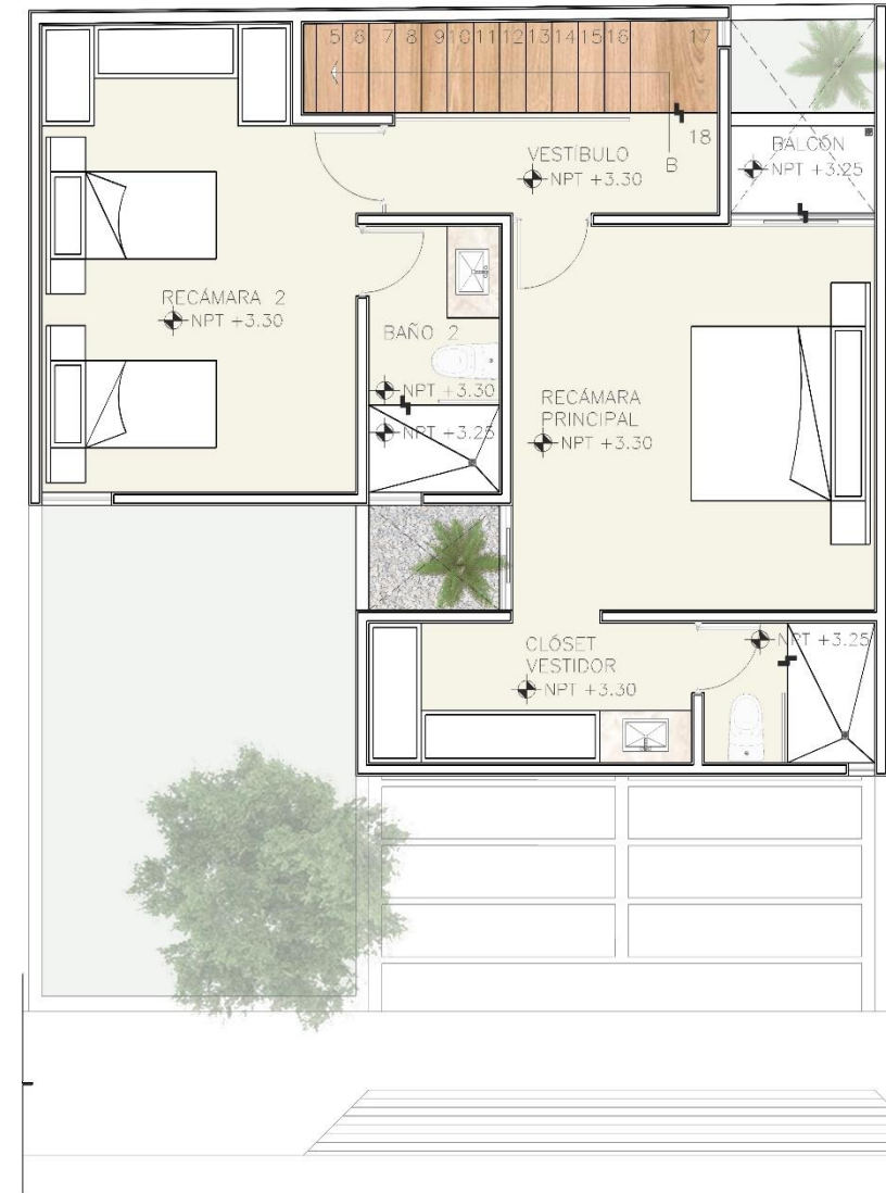
PLANTA ALTA
