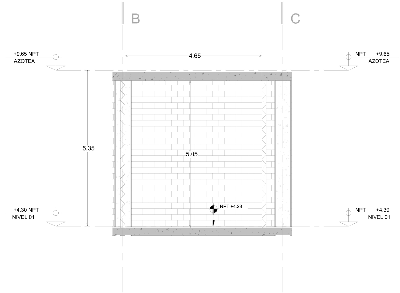
2 SECCIÓN A - A 1 : 75
