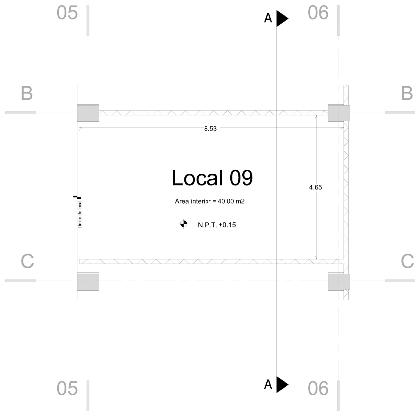
1 PLANTA LOCAL 09 1 : 75
