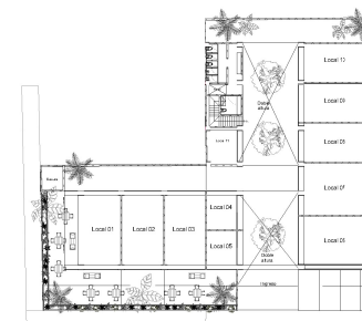
PLANTA UBICACIÓN 1 : 1000
