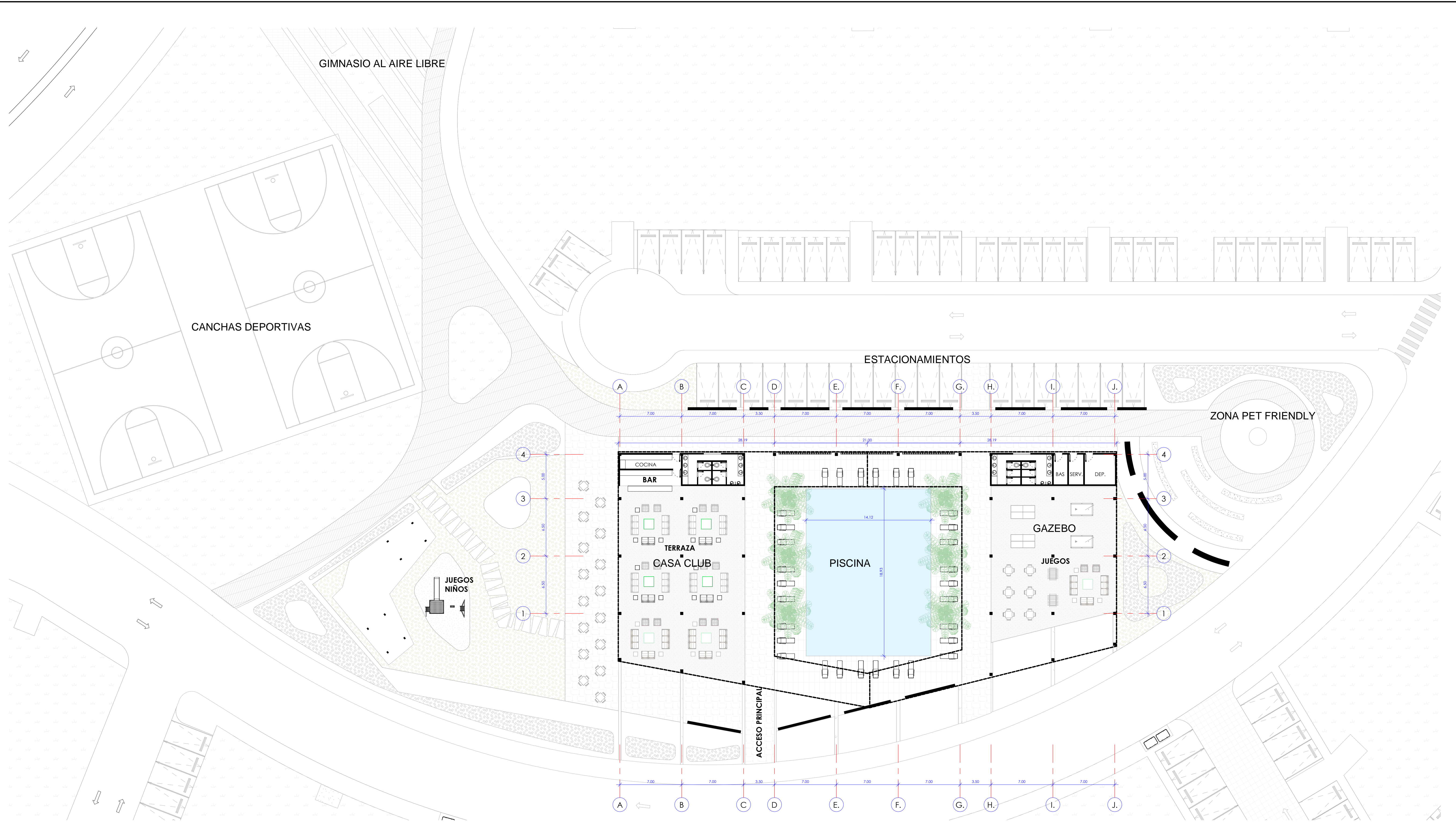
1 NIVEL 1 CASA CLUB 1 : 200
