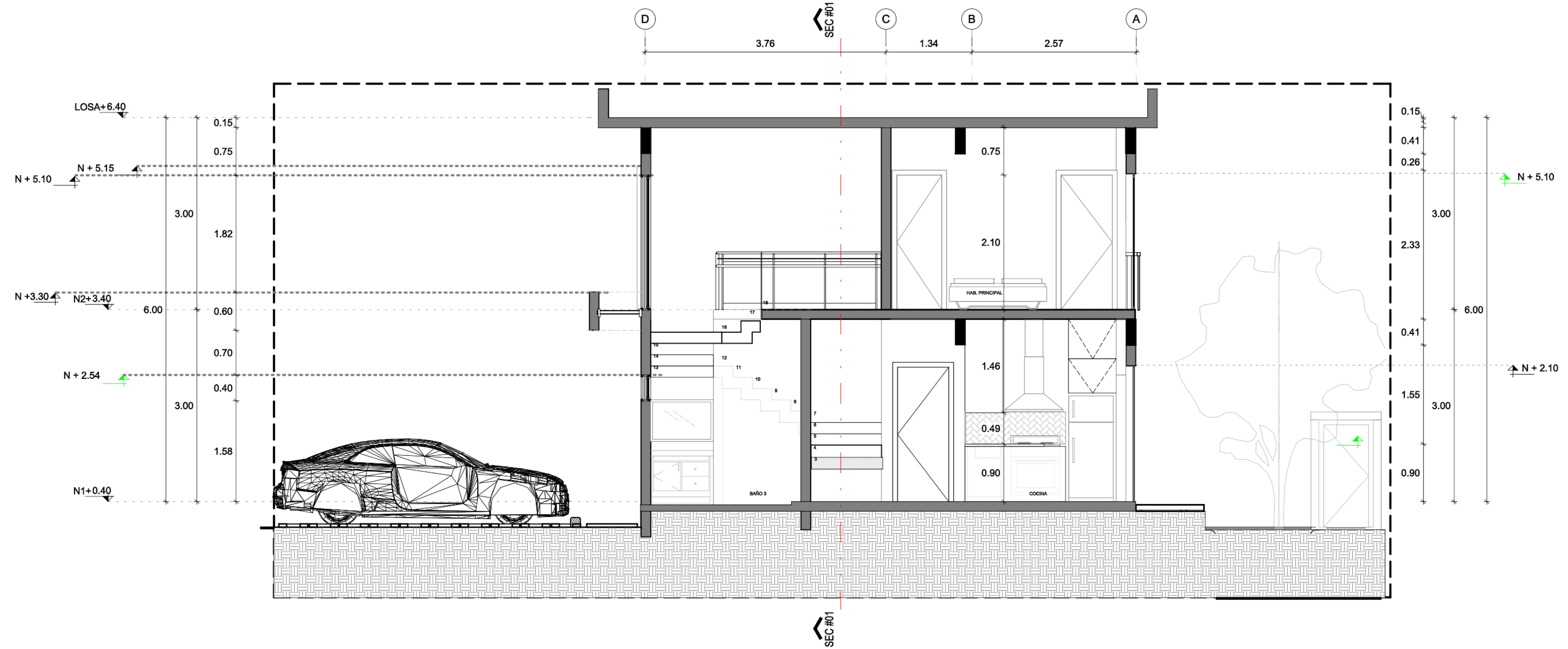
1 SECCION 1 ESC: 1 : 50
