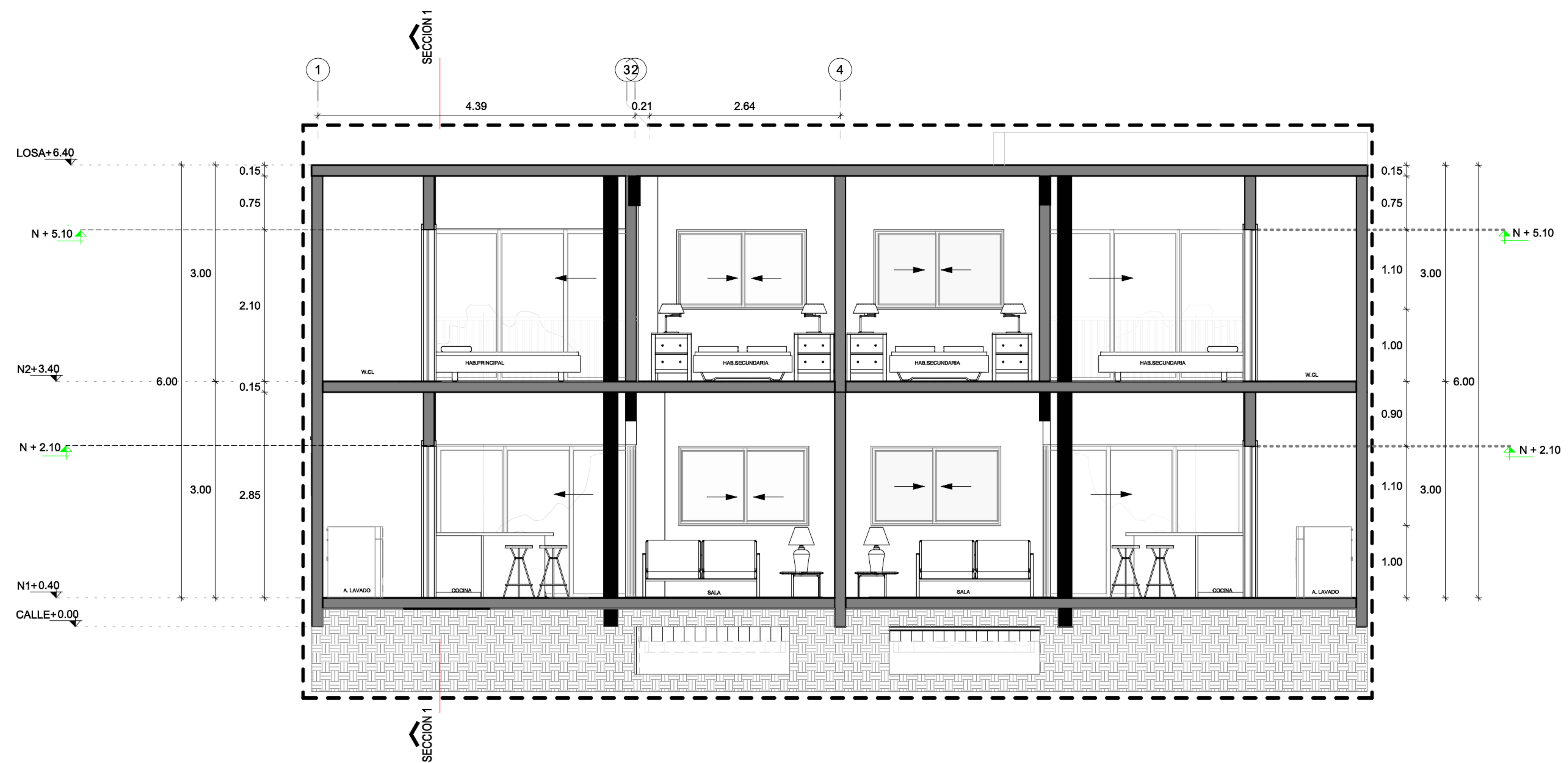
2 SECCION 2 ESC: 1 : 50
