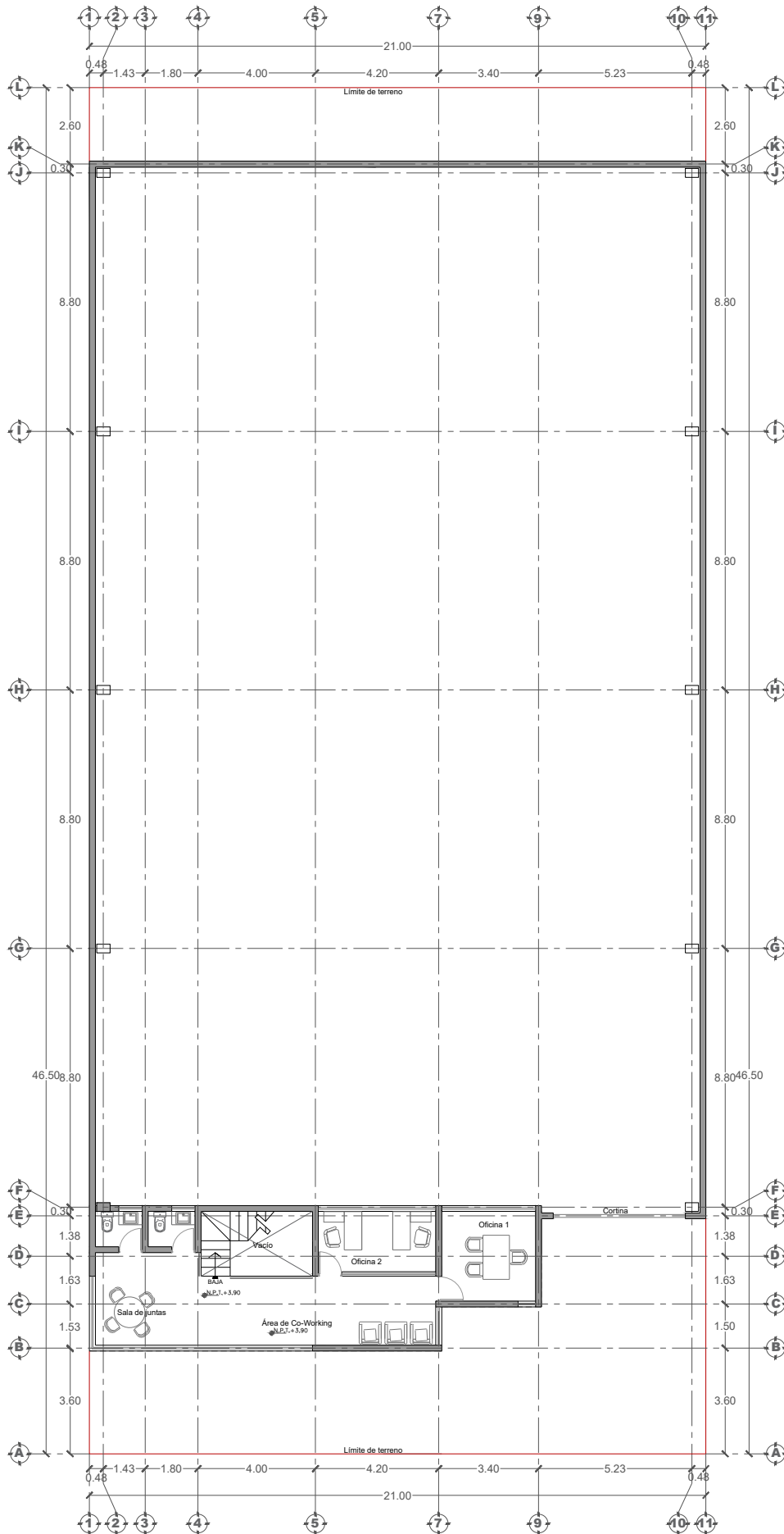
PLANTA ALTA ESCALA 1:100
