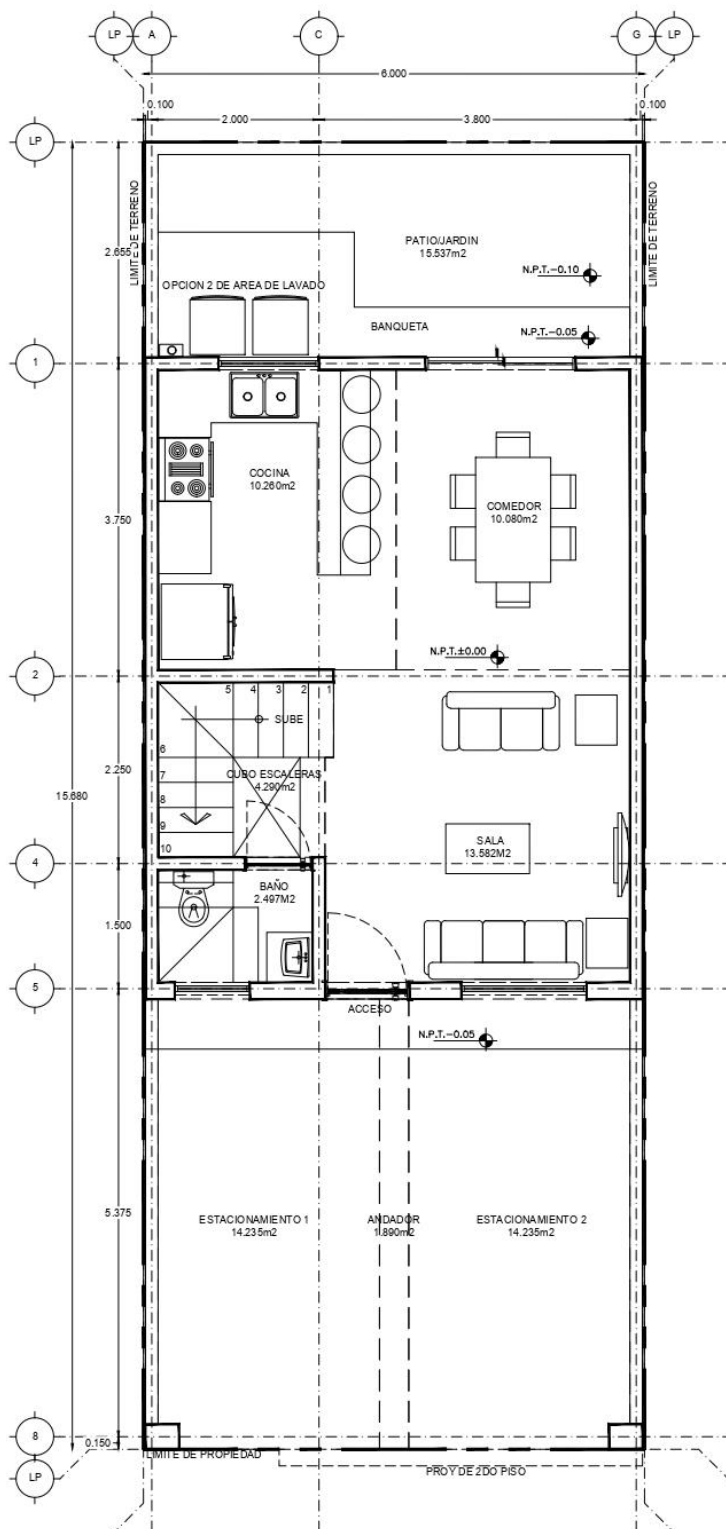
PLANTA BAJA
