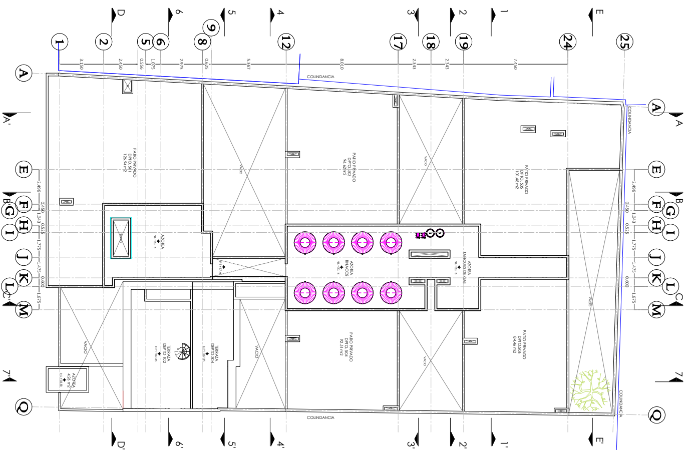
PLANTA DE AZOTEA / SERVICIOS N+20.16 TANQUES DE GAS Y TINACOS
