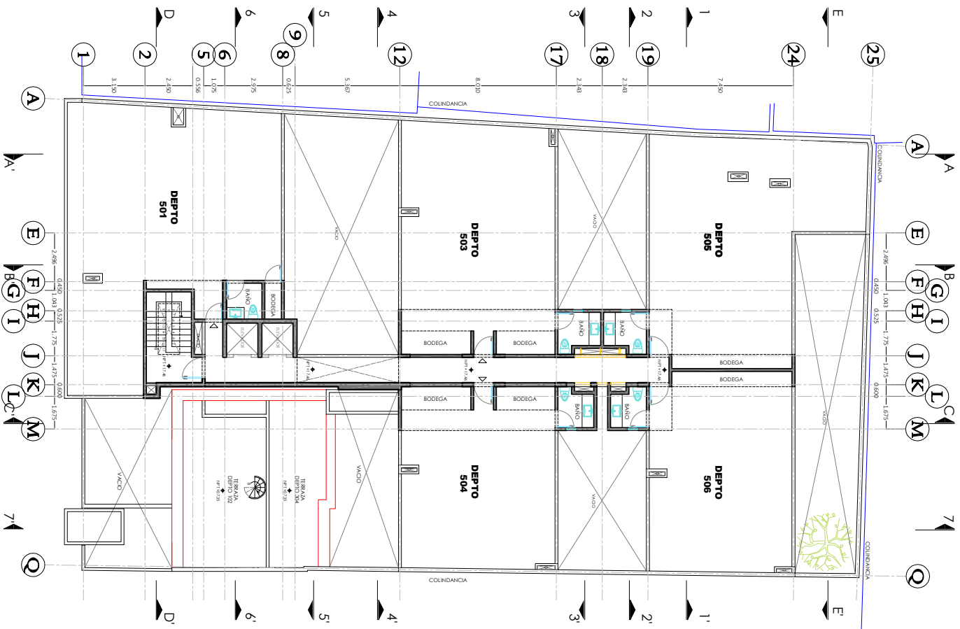
PLANTA DE AZOTEAS / PATIOS N+17.46 PATIOS PRIVADOS
