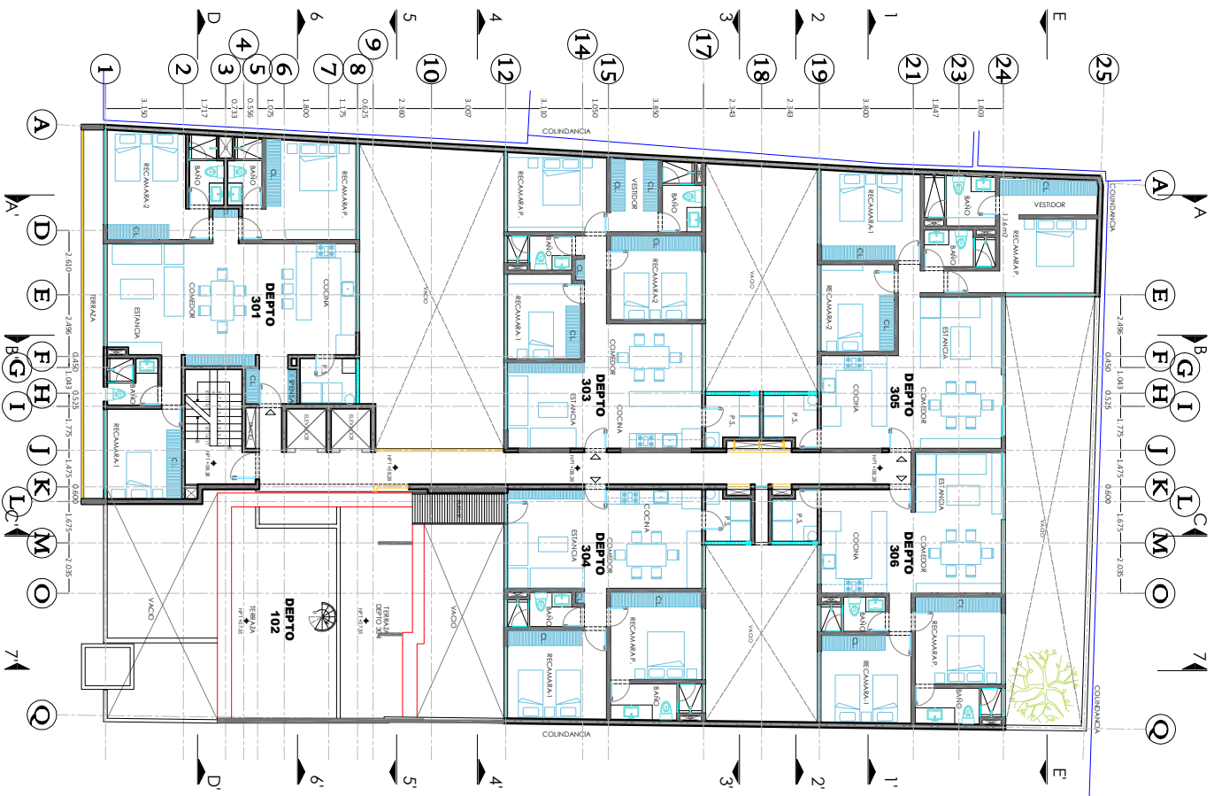
PLANTA 3° NIVEL N+08.28 DEPARTAMENTOS
