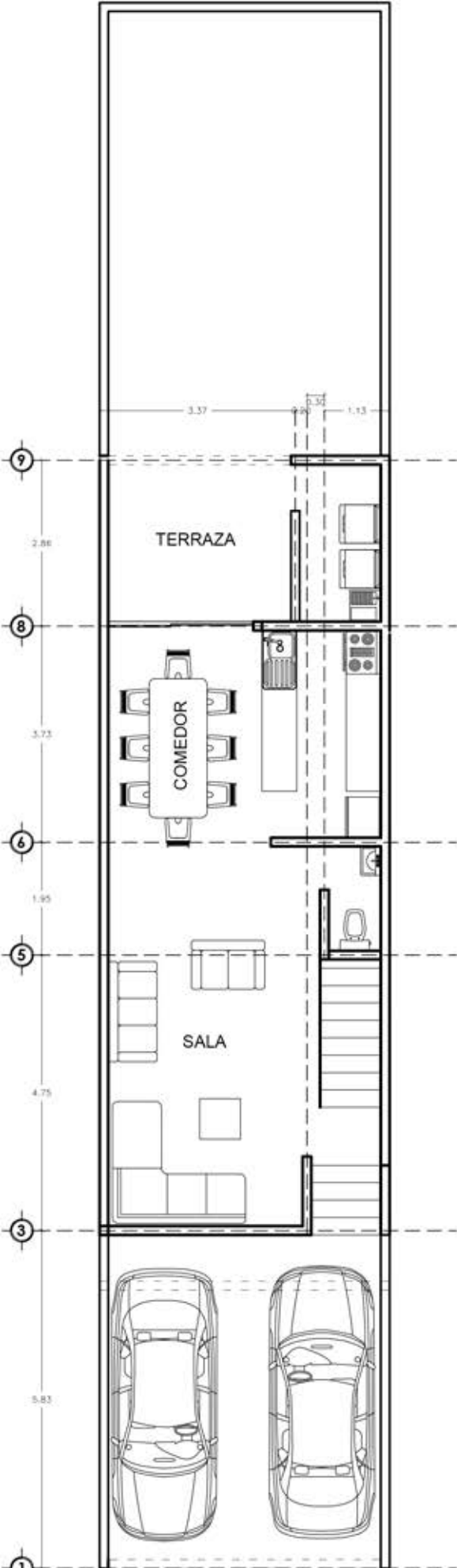
PLANTA BAJA
