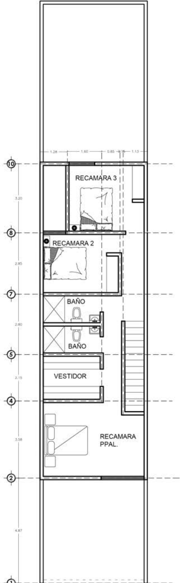
PLANTA ALTA
