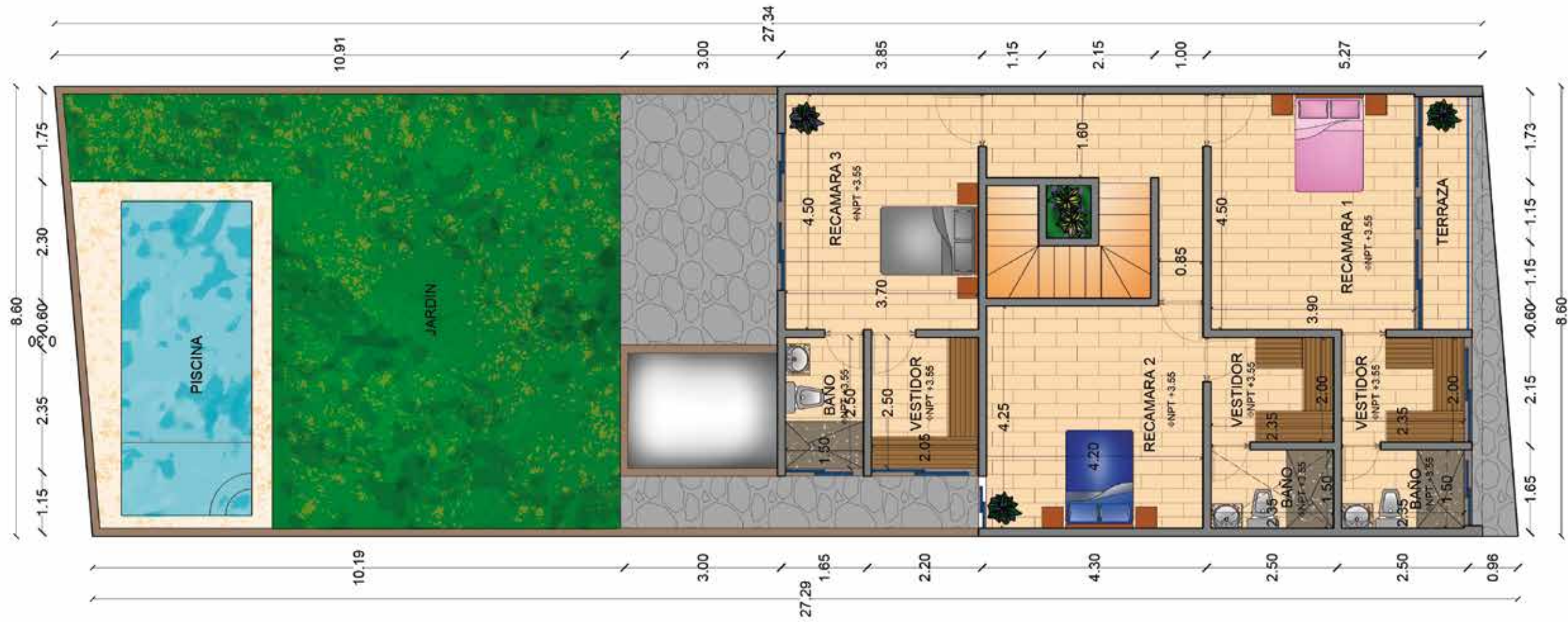
PLANTA ALTA
