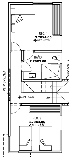
PLANTA ALTA ÁREA 54.53 M2
