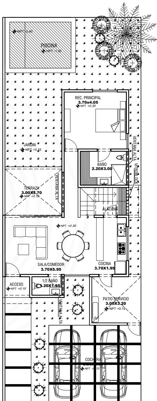
PLANTA BAJA ÁREA 72.54 M2 TOTAL 127.07 M2
