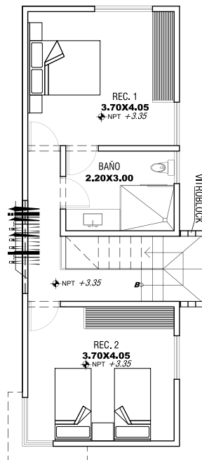
PLANTA ALTA ÁREA 54.53 M2
