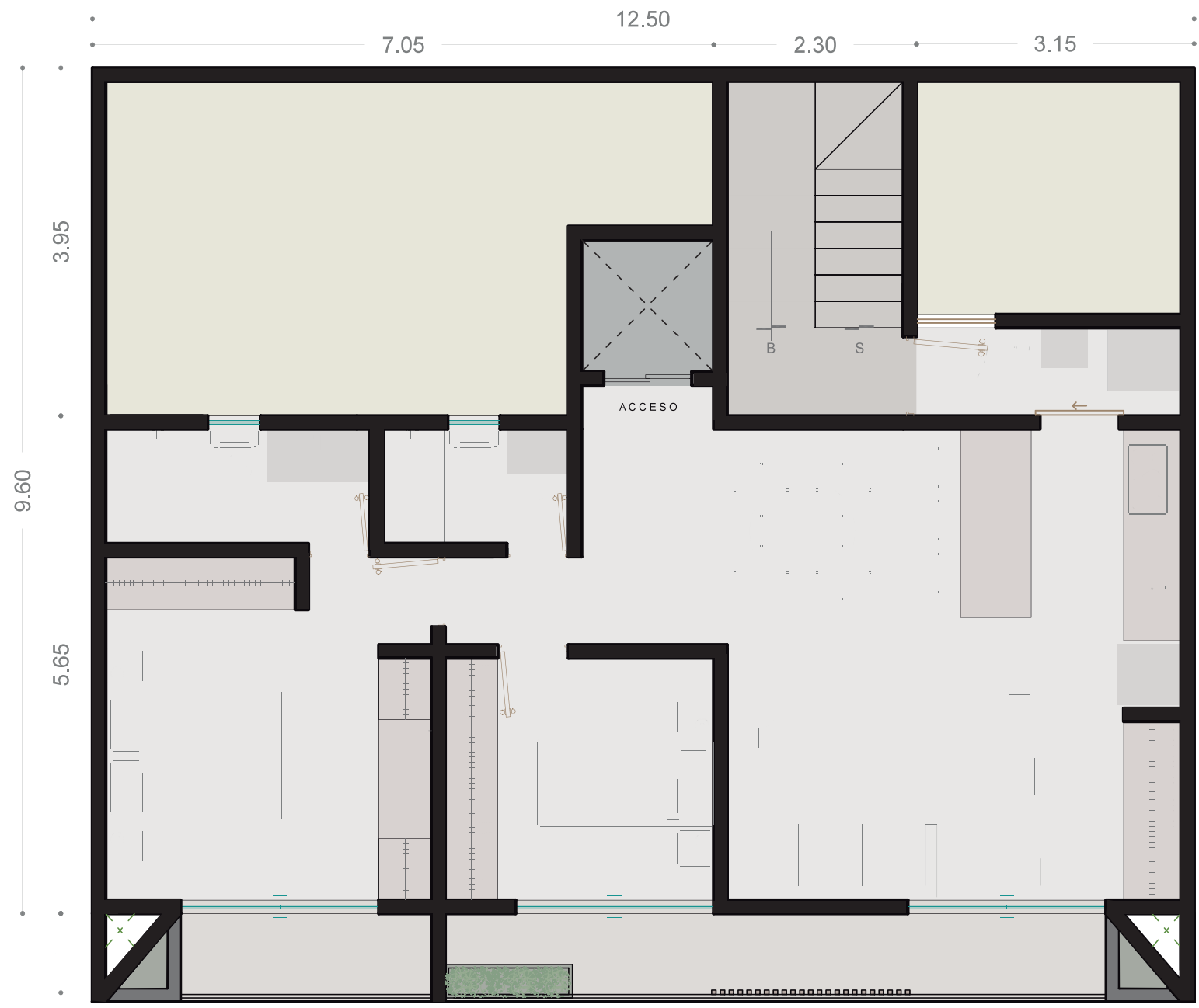
DEPARTAMENTO TIPO
