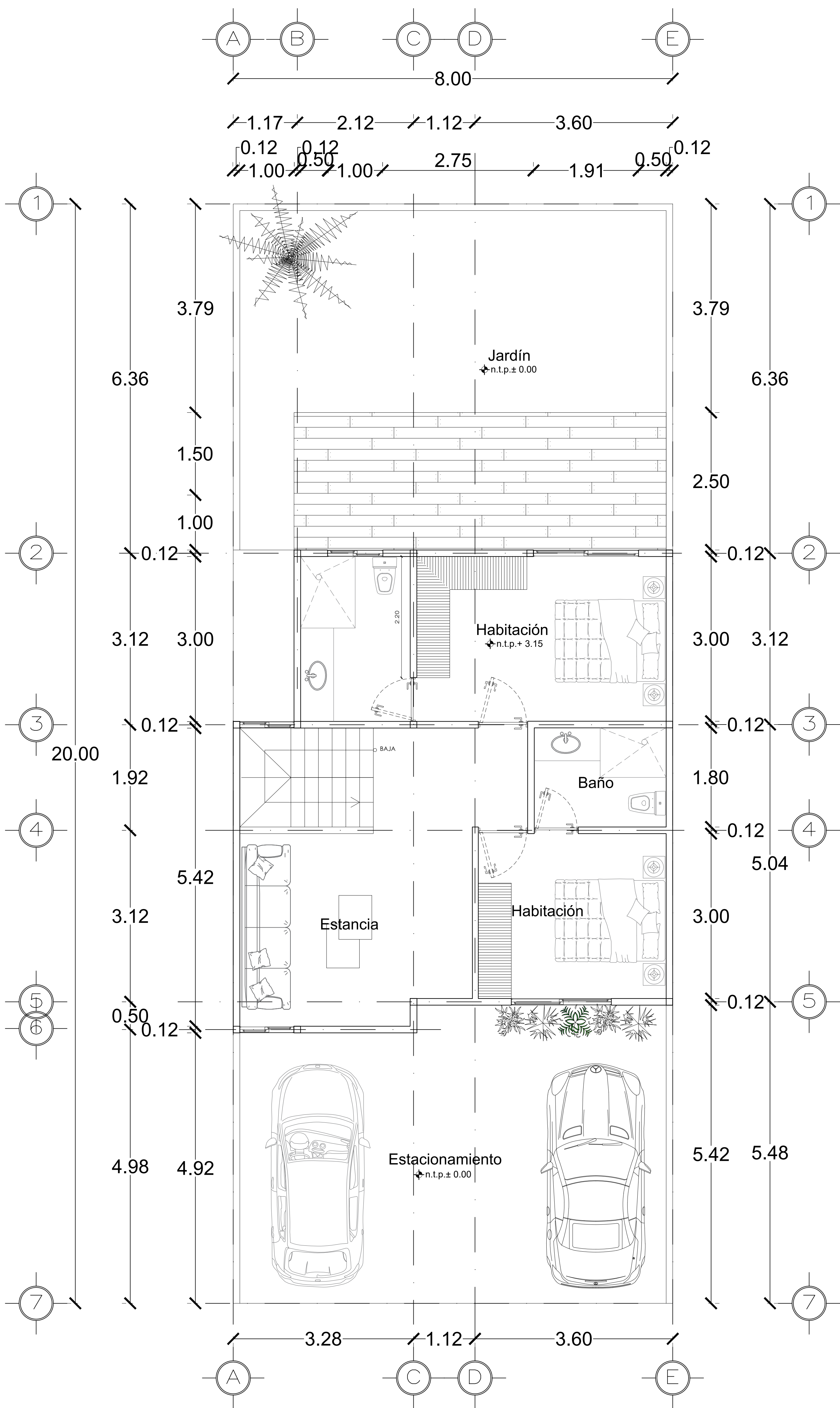
PRIMER NIVEL
