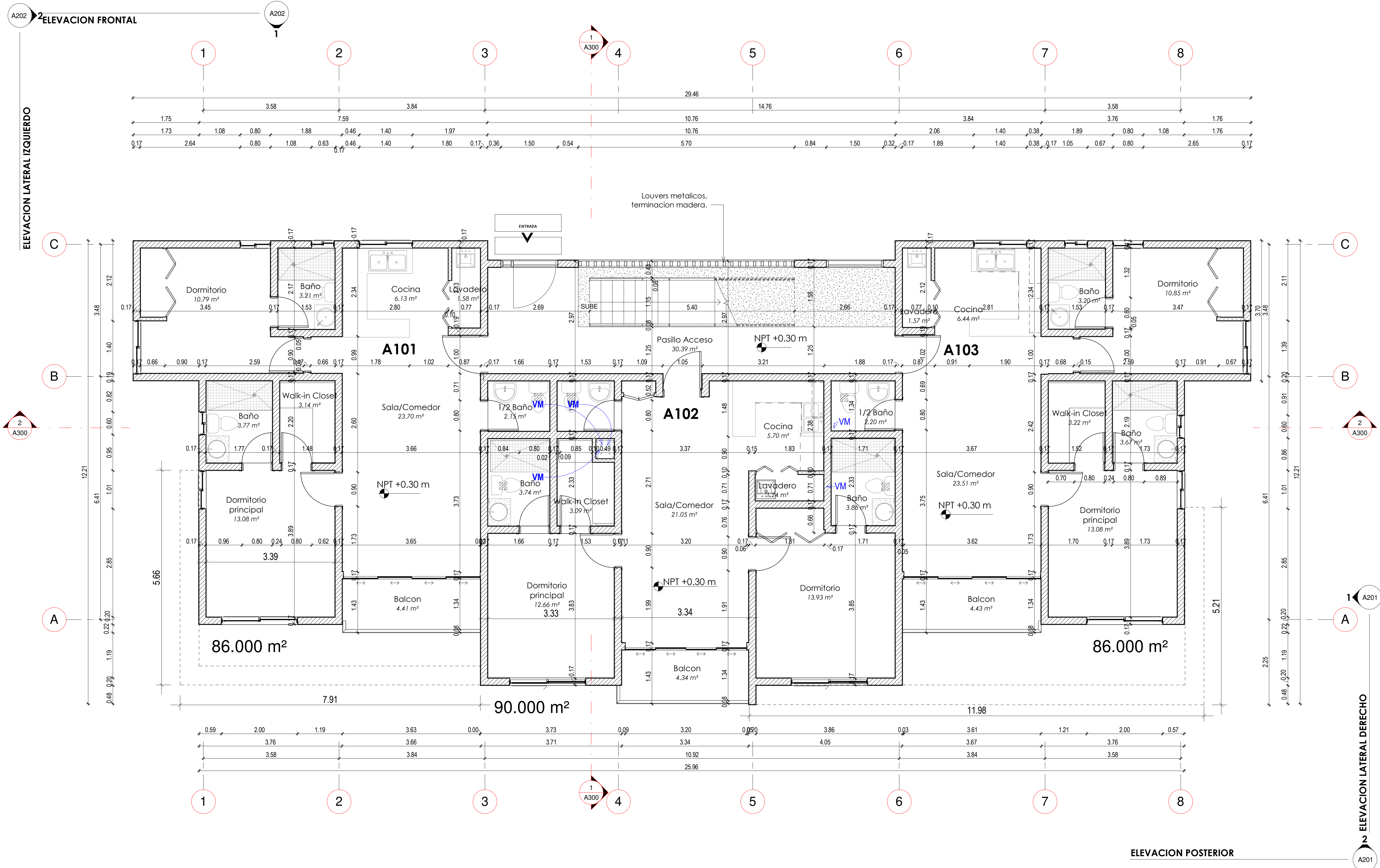
1 PLANTA ARQUITECTÓNICA DIMENSIONADA - TIPO A A111 esc: 1 : 50
