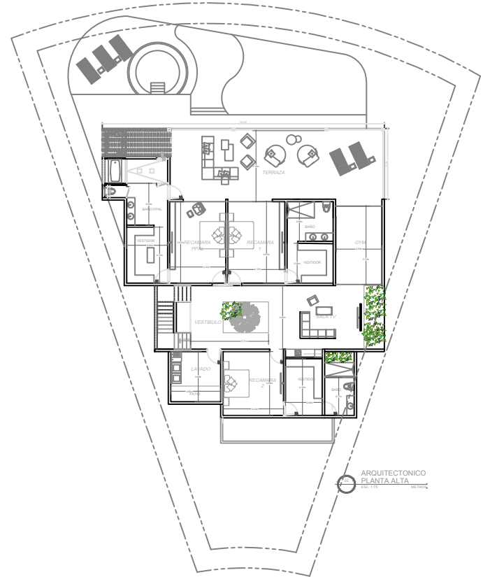
PLANTA ALTA
