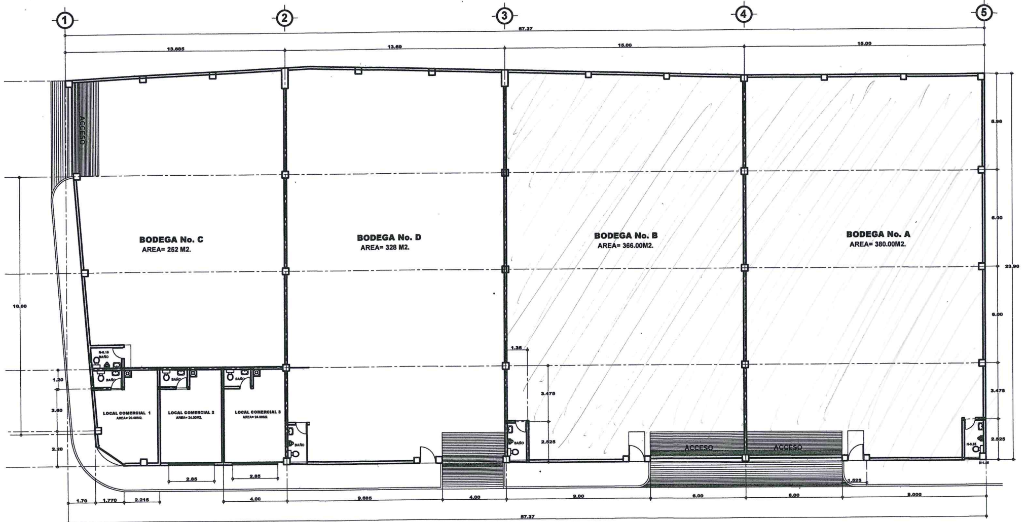
PLANTA BAJA
