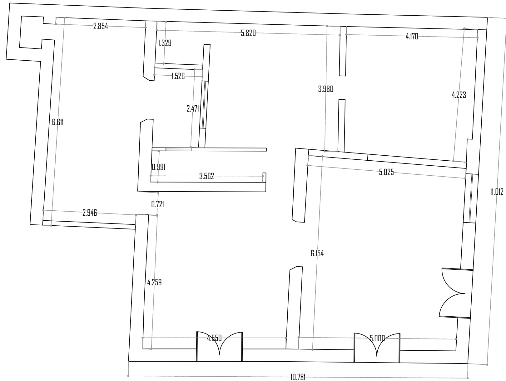
LEVANTAMIENTO CASA CALLE 12 Y CORREGIDORA
