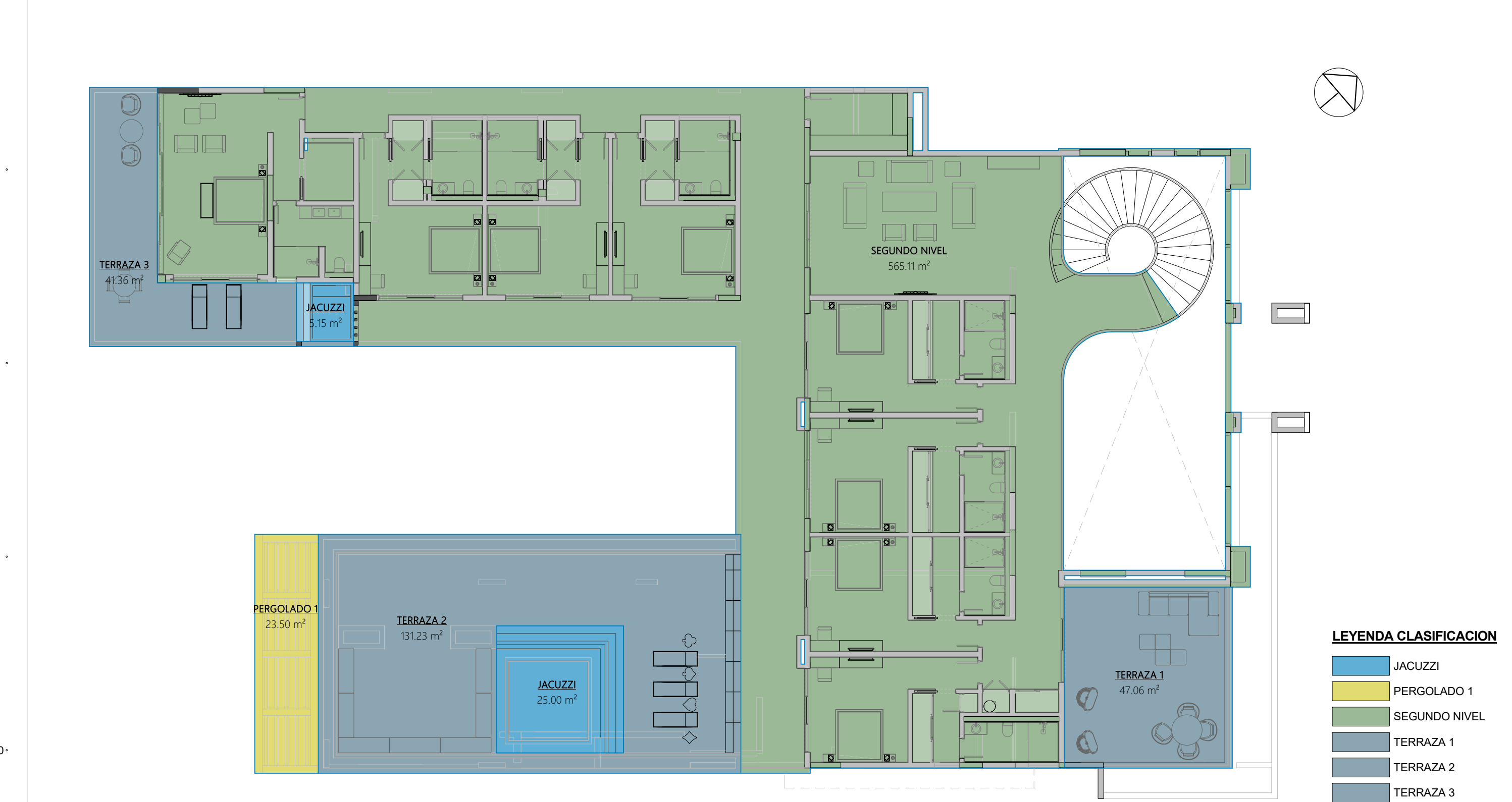
02 PLANTA ARQUITECTONICA 2DO NIVEL ESC 1: 150
