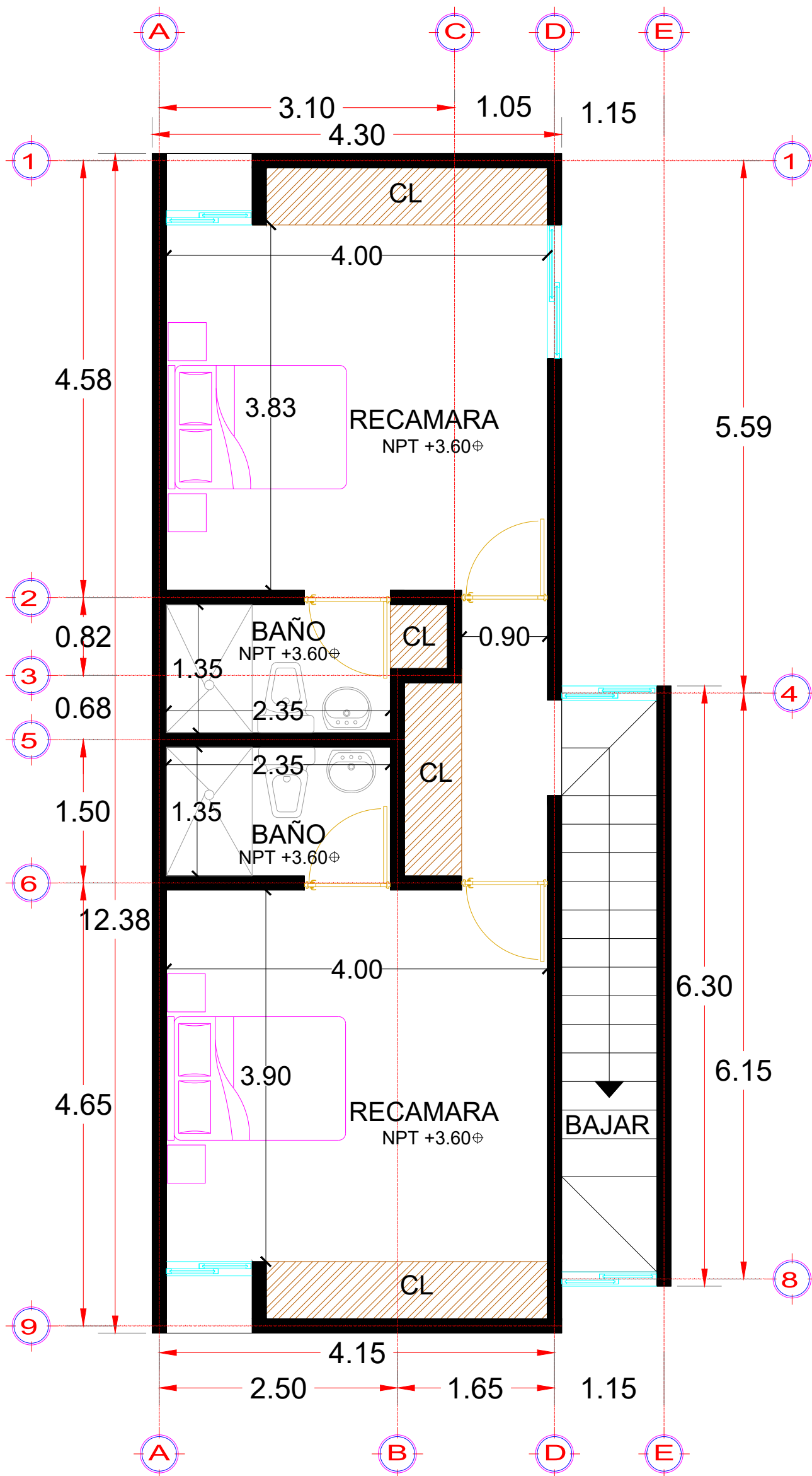
PLANTA ALTA
